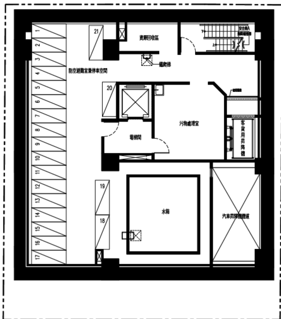
地下室貳層平面圖(建照圖)
