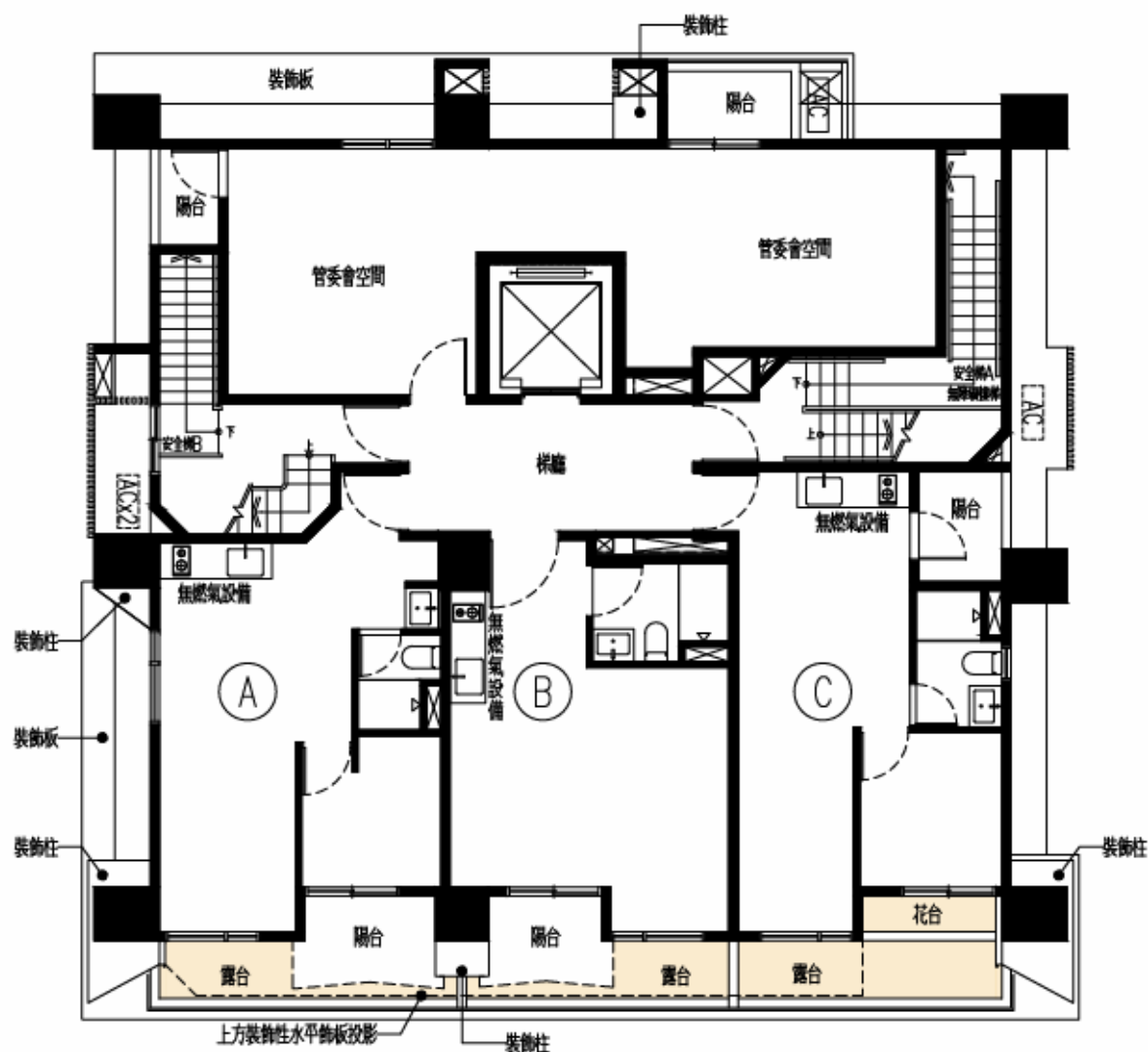
貳層平面圖(建照圖)
