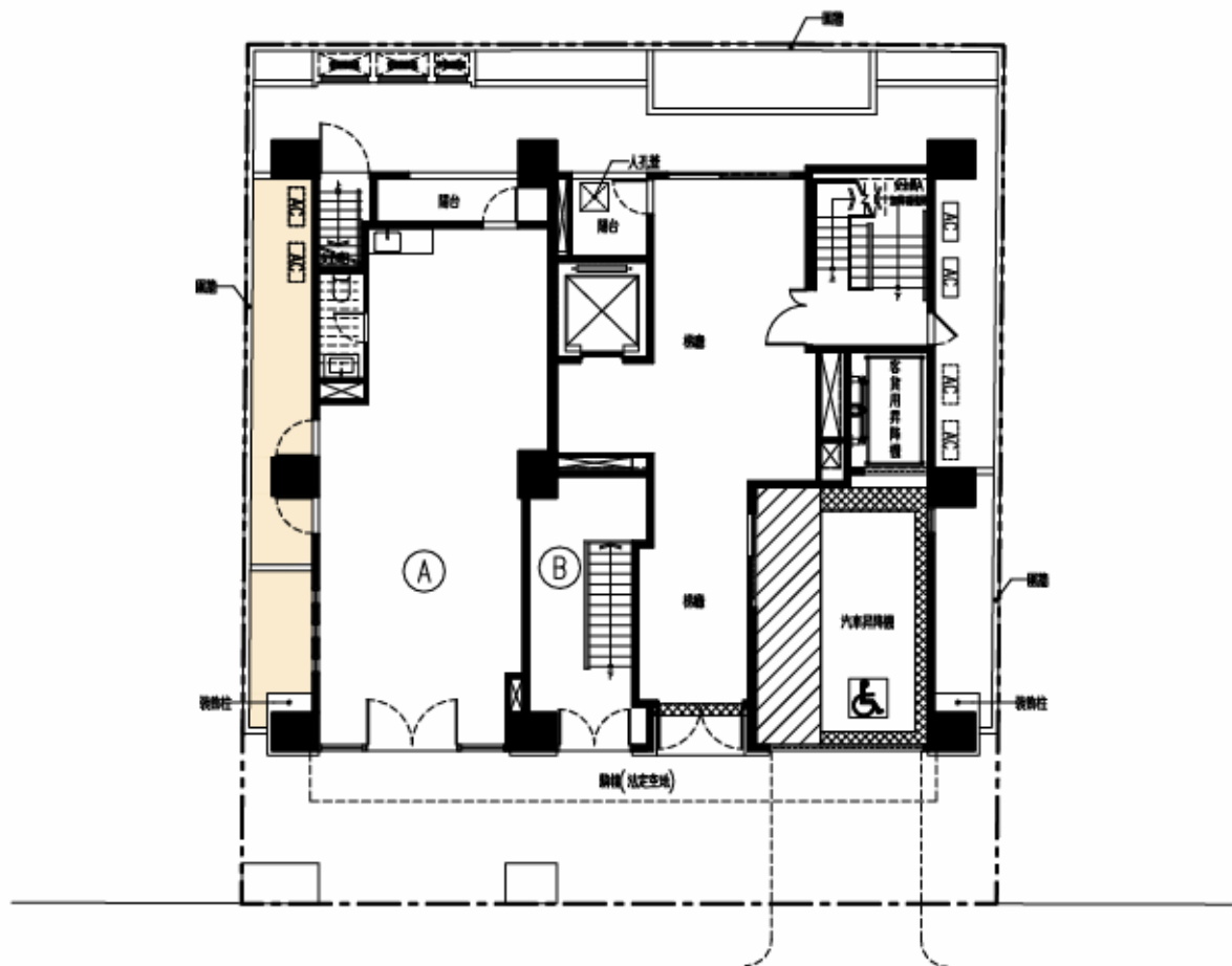
壹層平面圖(建照圖)
