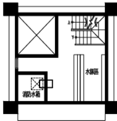
屋突貳層平面圖(建照圖)
