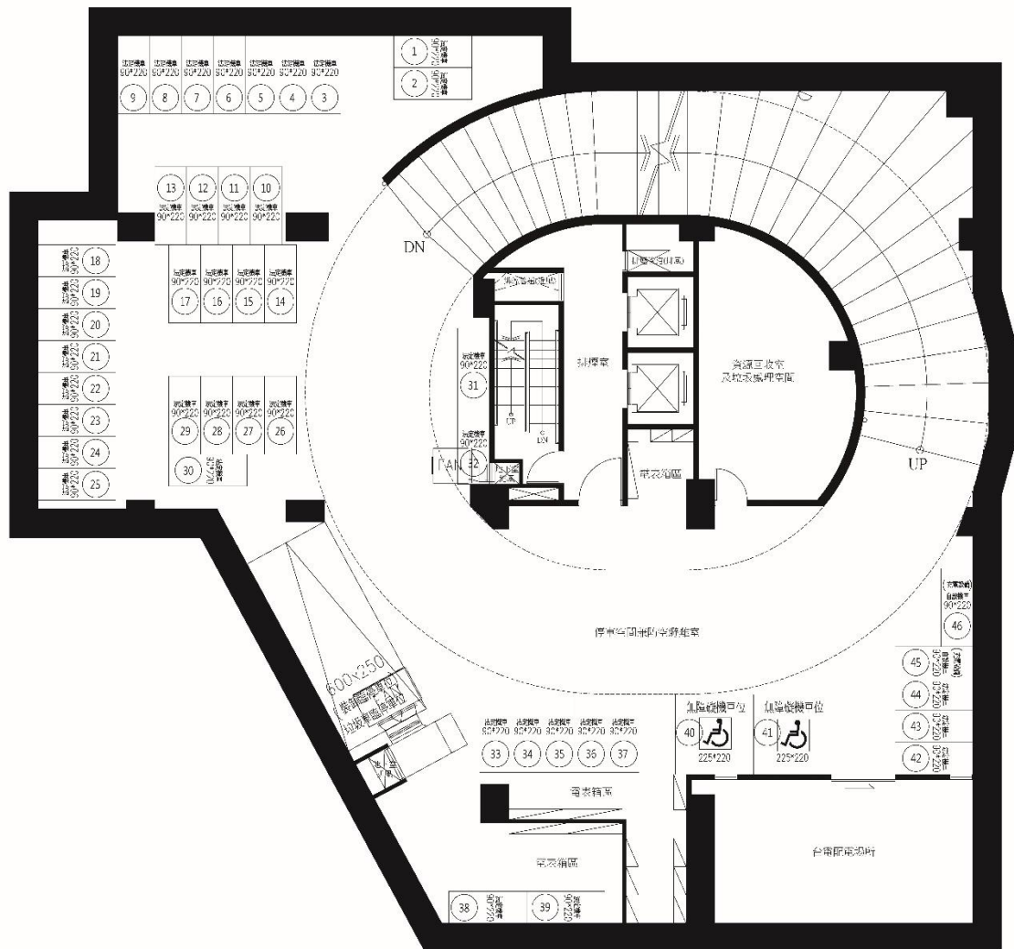
地下一層平面圖 南海御景
