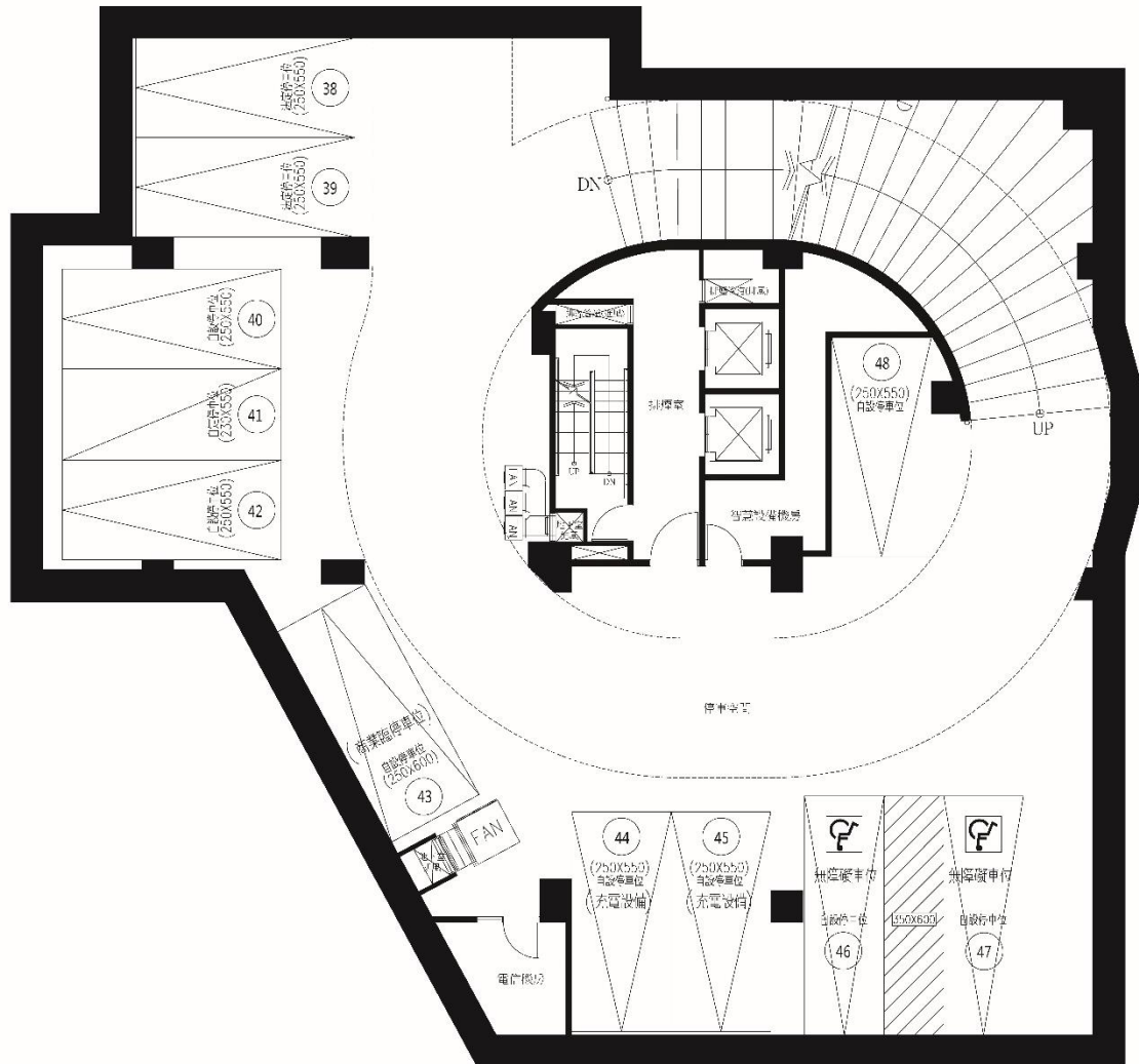
地下二層平面圖 南海御景
