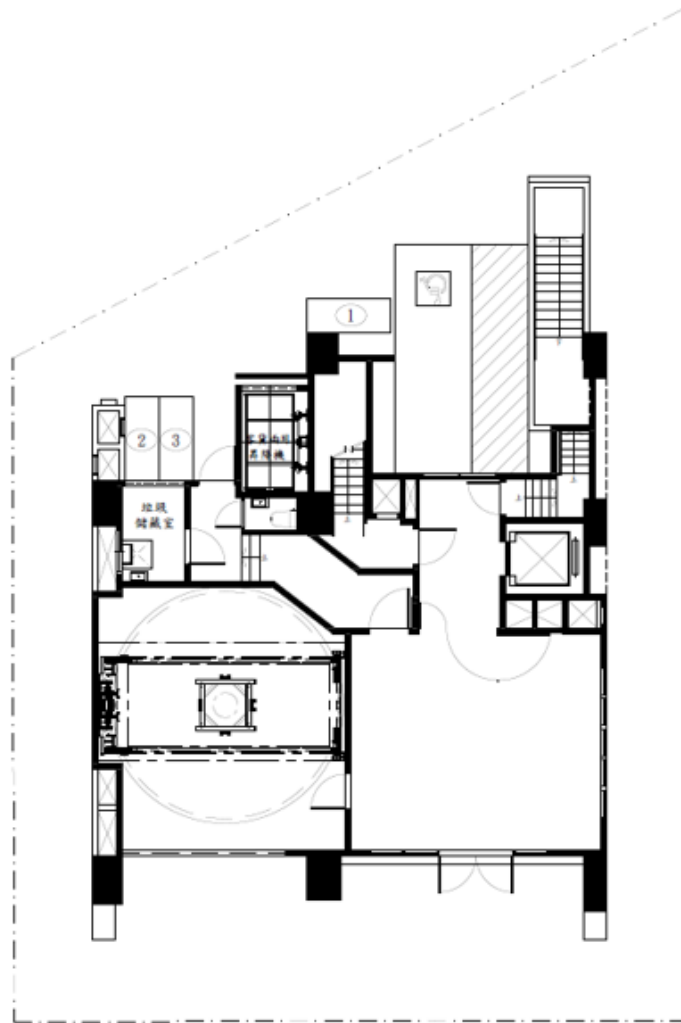
一層平面圖
