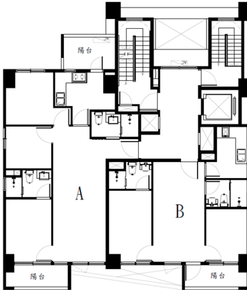
十層平面圖
