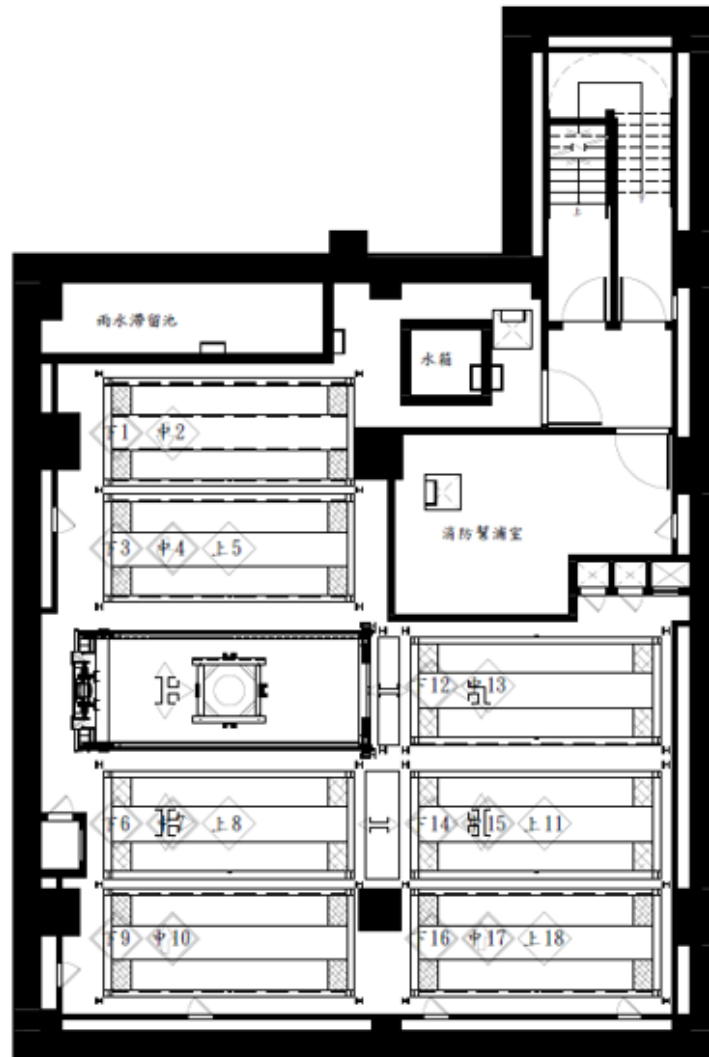
地下二層平面圖
