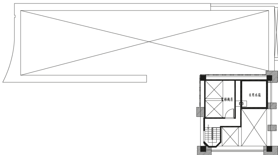
屋突三層平面圖
