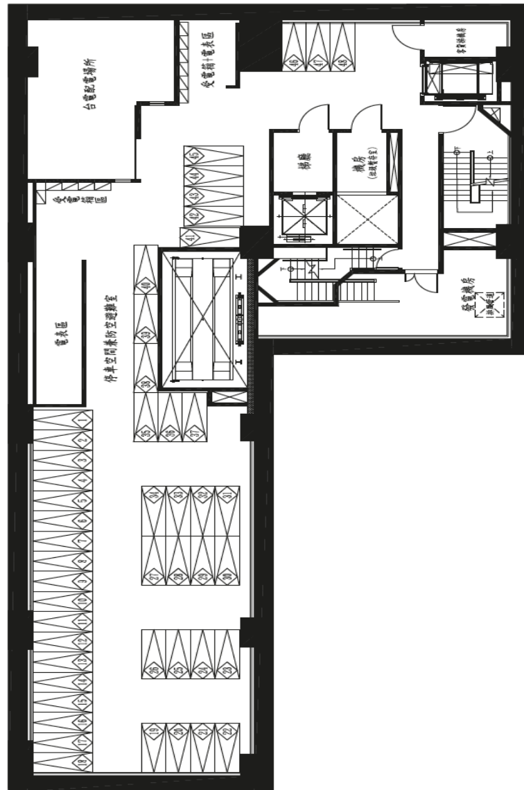
地下壹層平面圖
