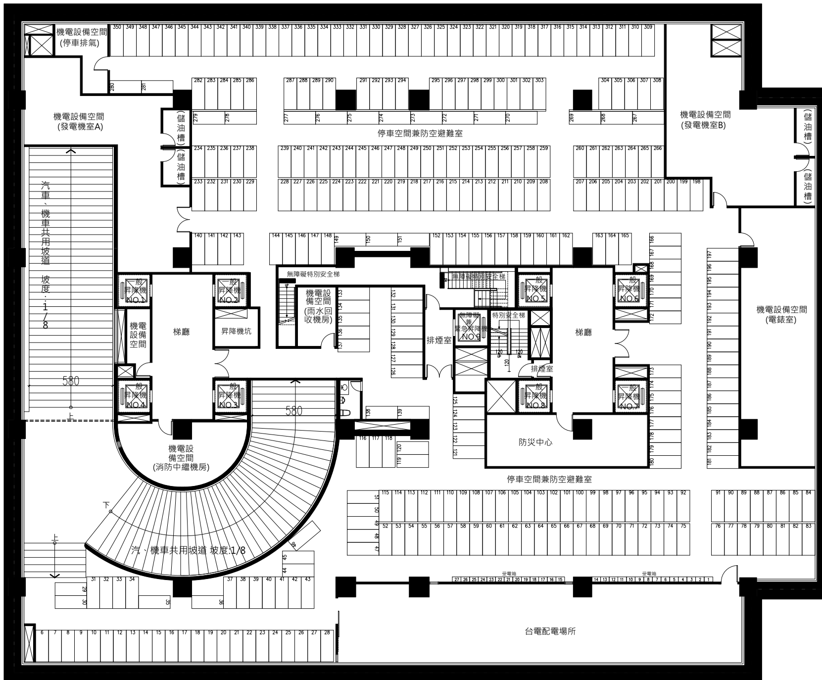
(建照圖) 地下一層平面圖
