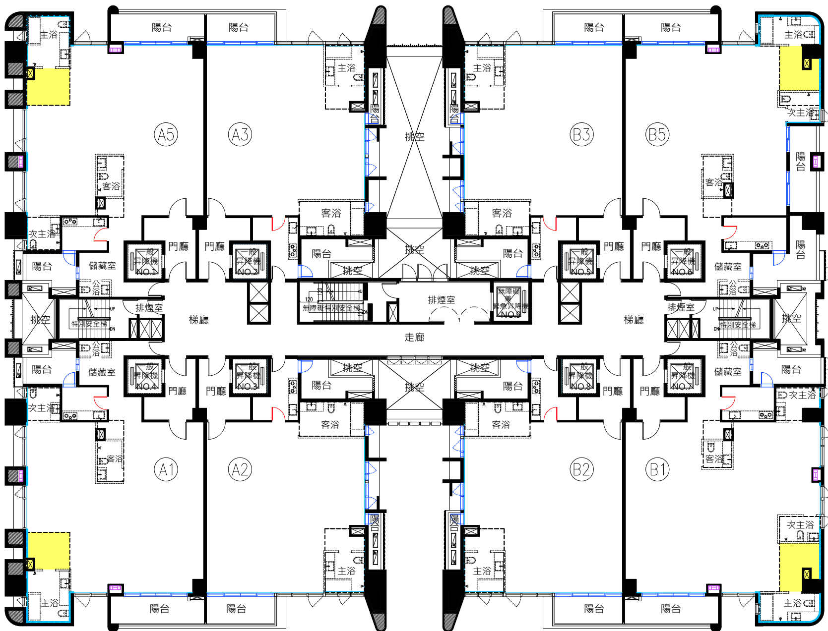
(建照圖) 十四至十七層平面圖
