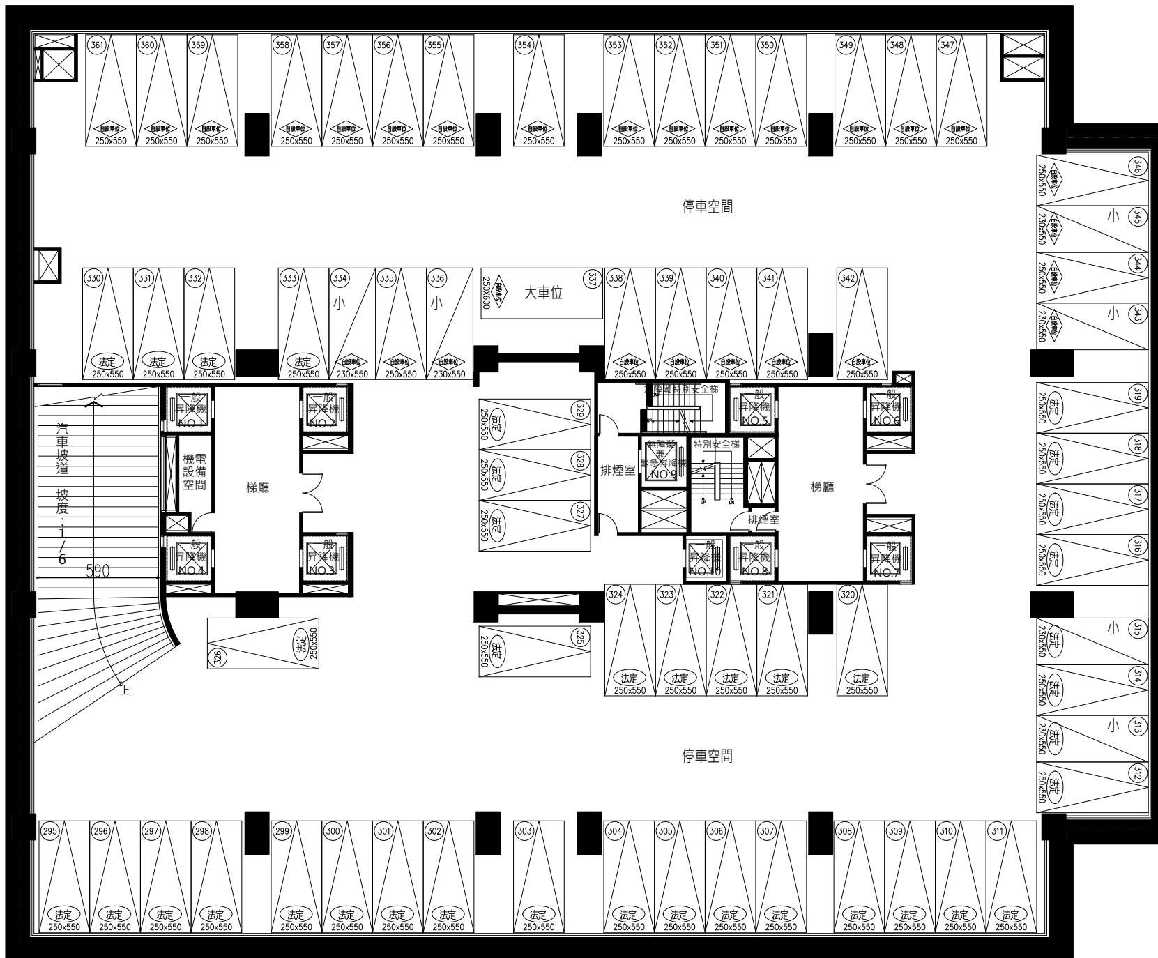
(建照圖) 地下七層平面圖
