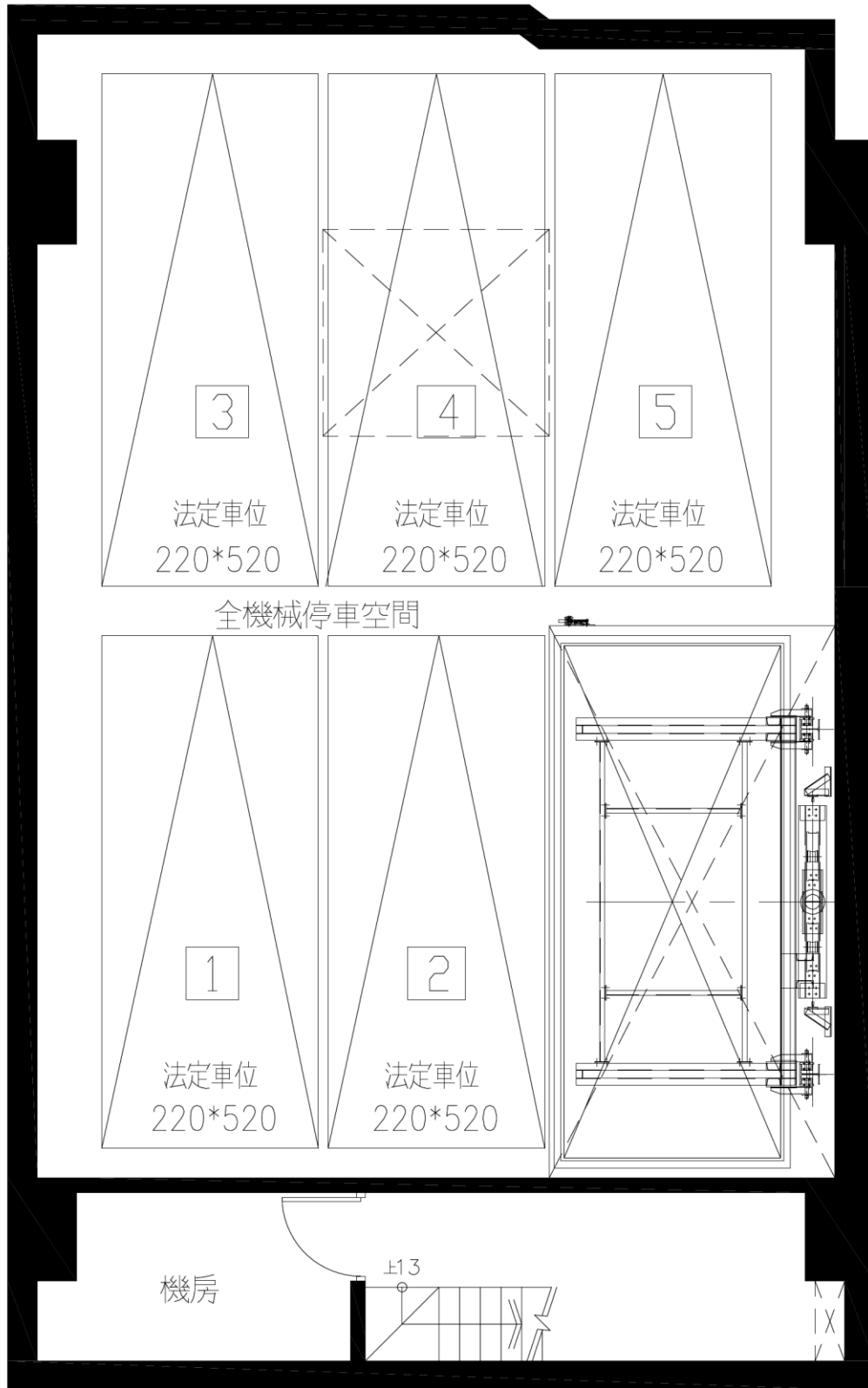
地下二層平面圖
