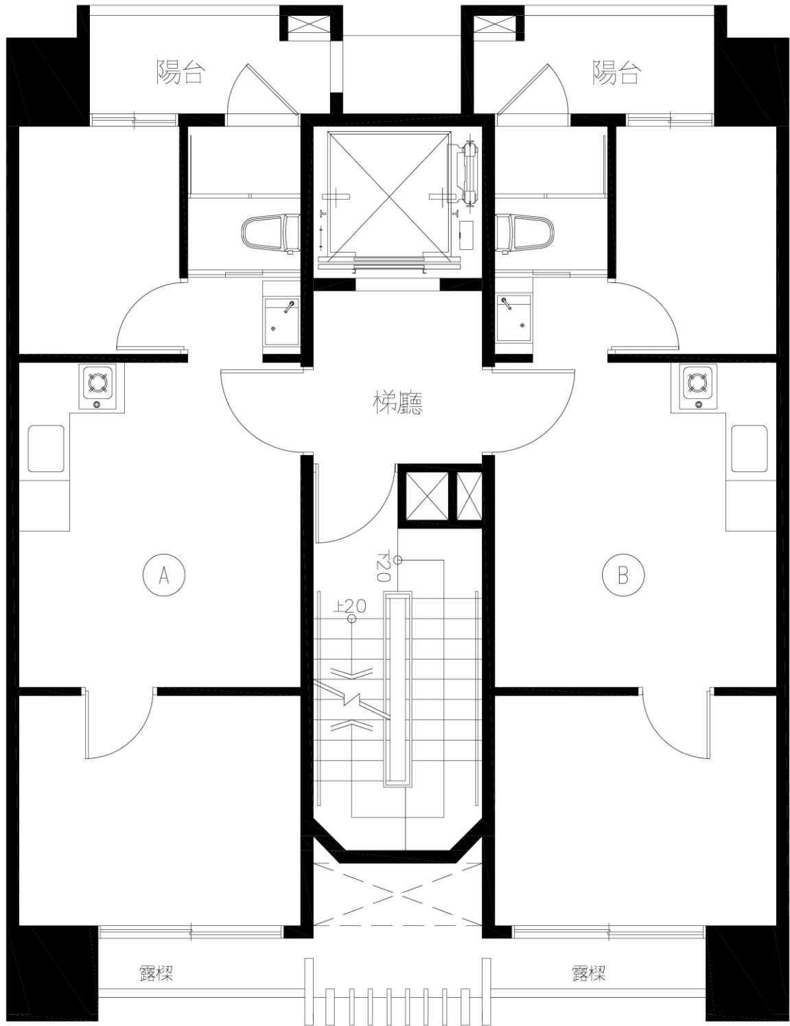
二層至六層平面圖
