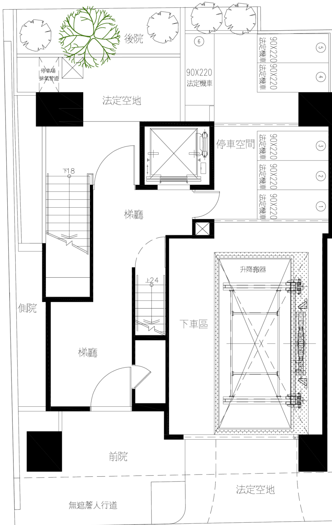
一層平面圖
