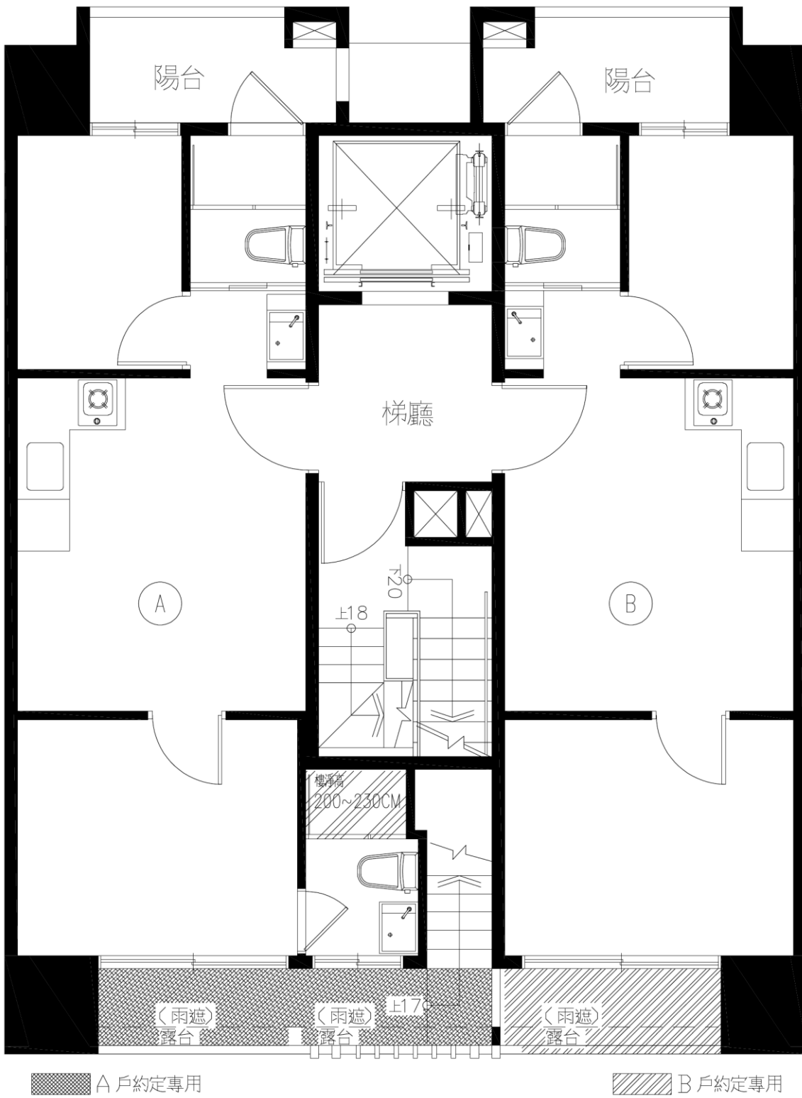
七層平面圖
