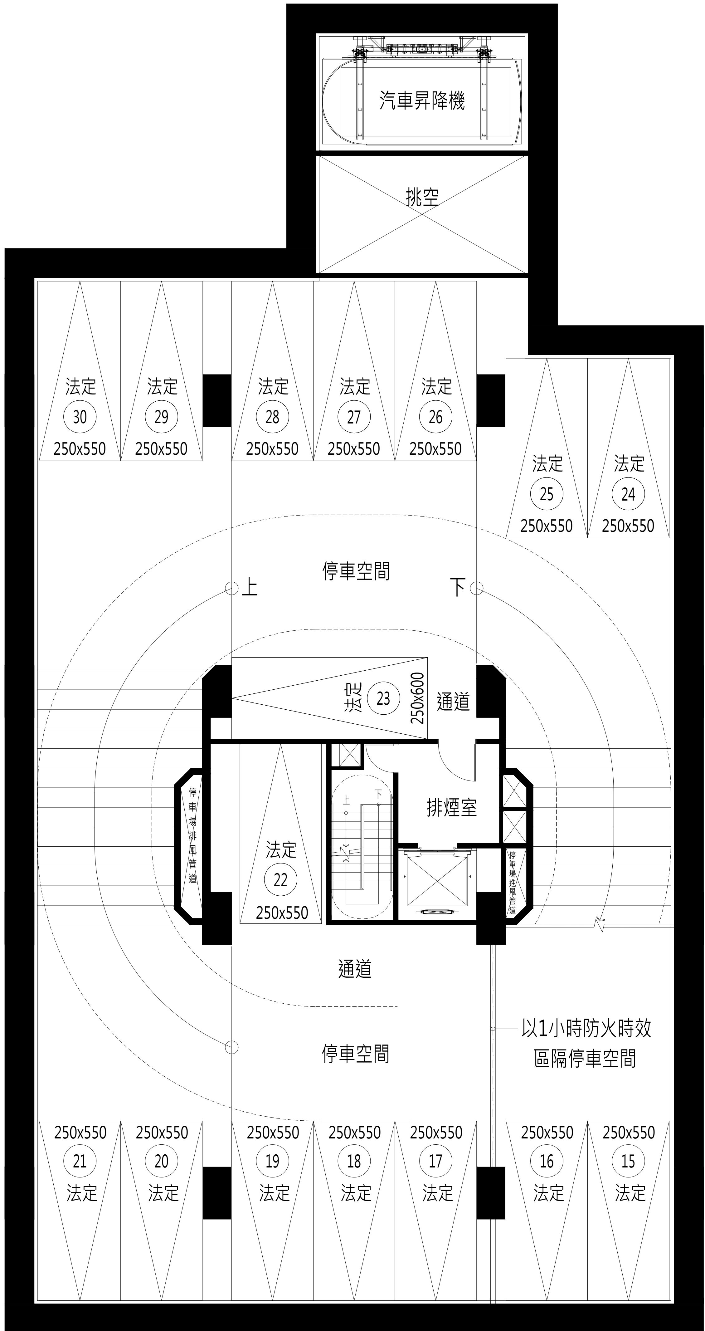
地下五層平面圖
