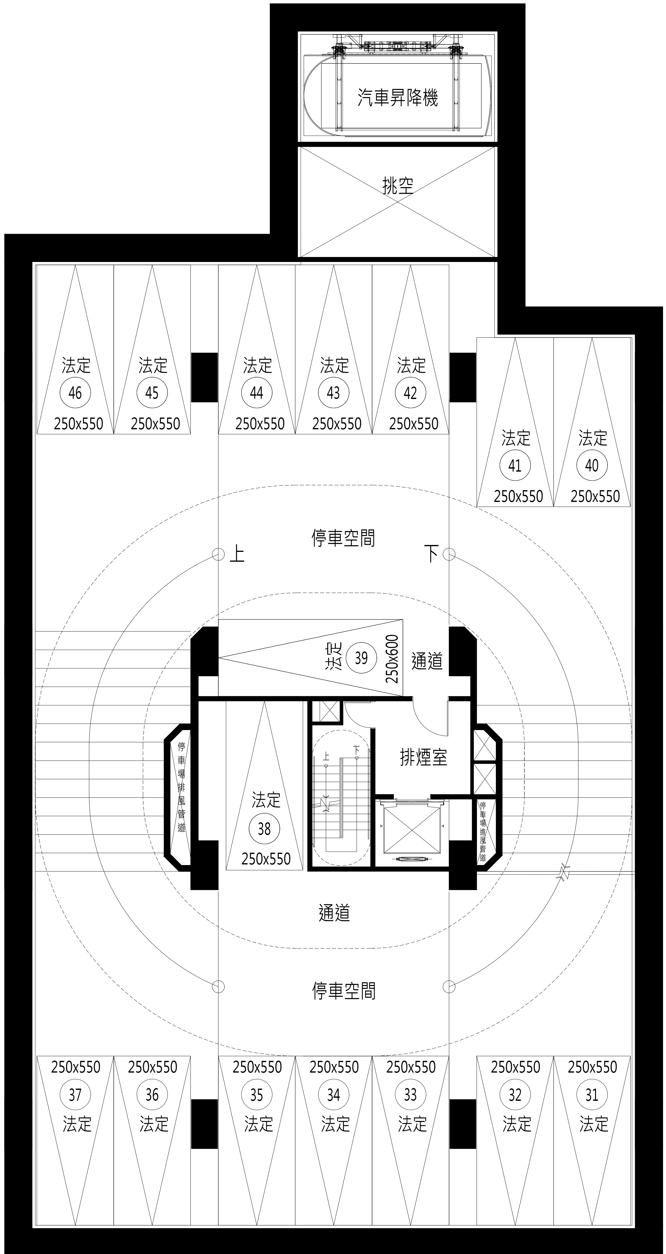
地下四層平面圖
