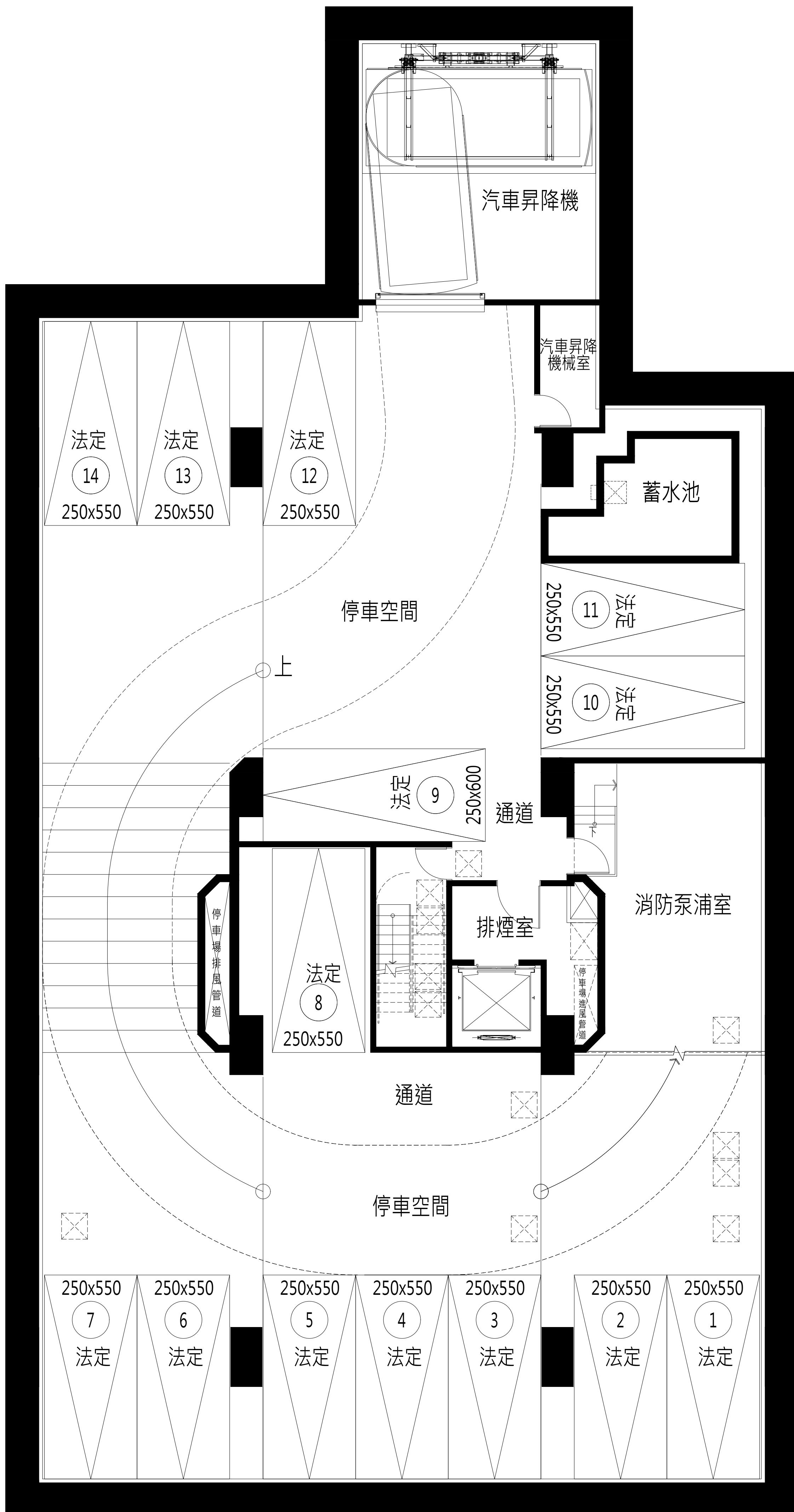
地下六層平面圖
