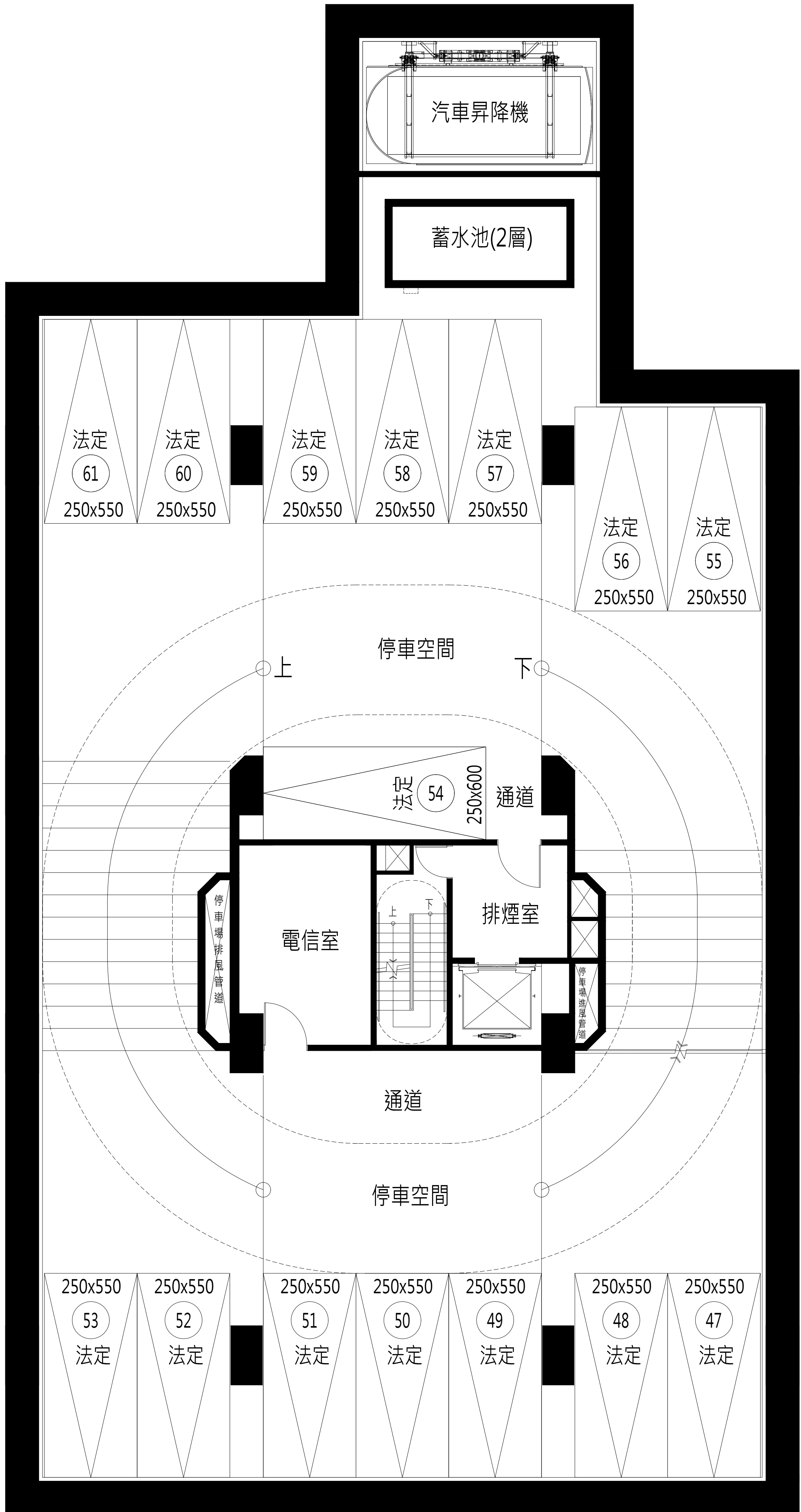
地下三層平面圖
