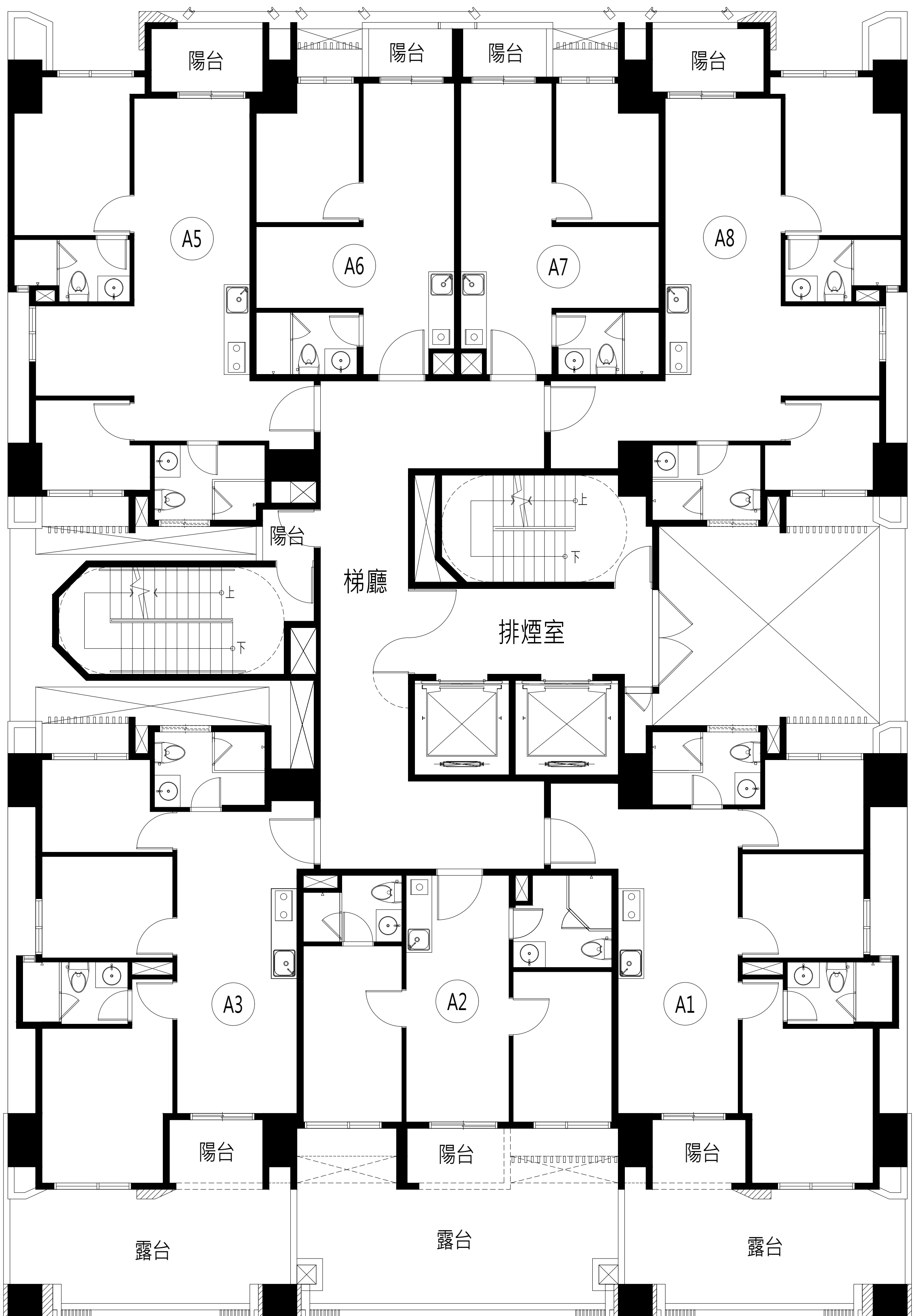
三樓平面圖
