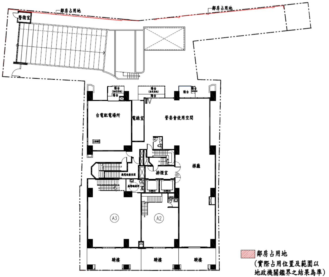
壹樓平面圖
