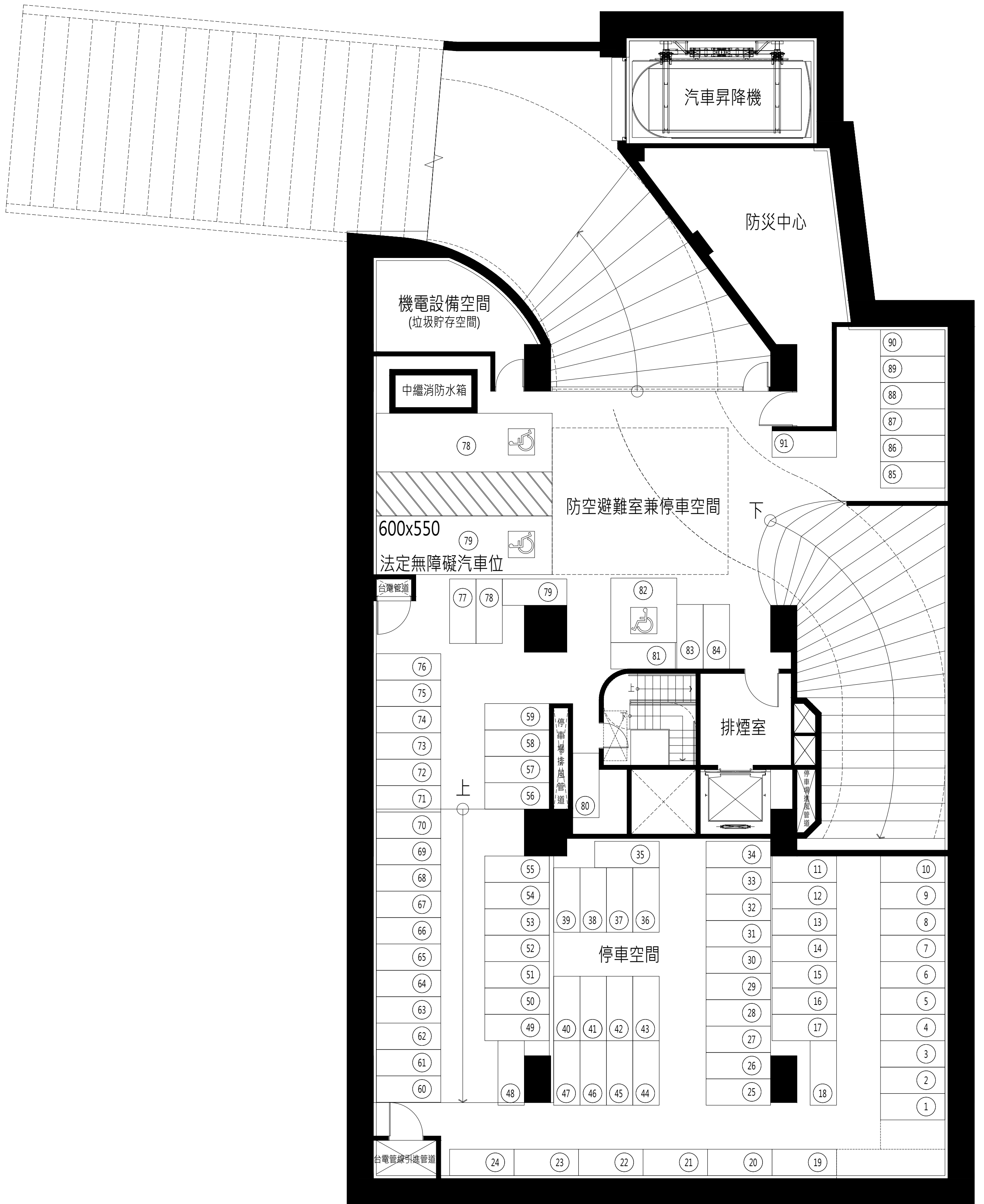
地下一層平面圖
