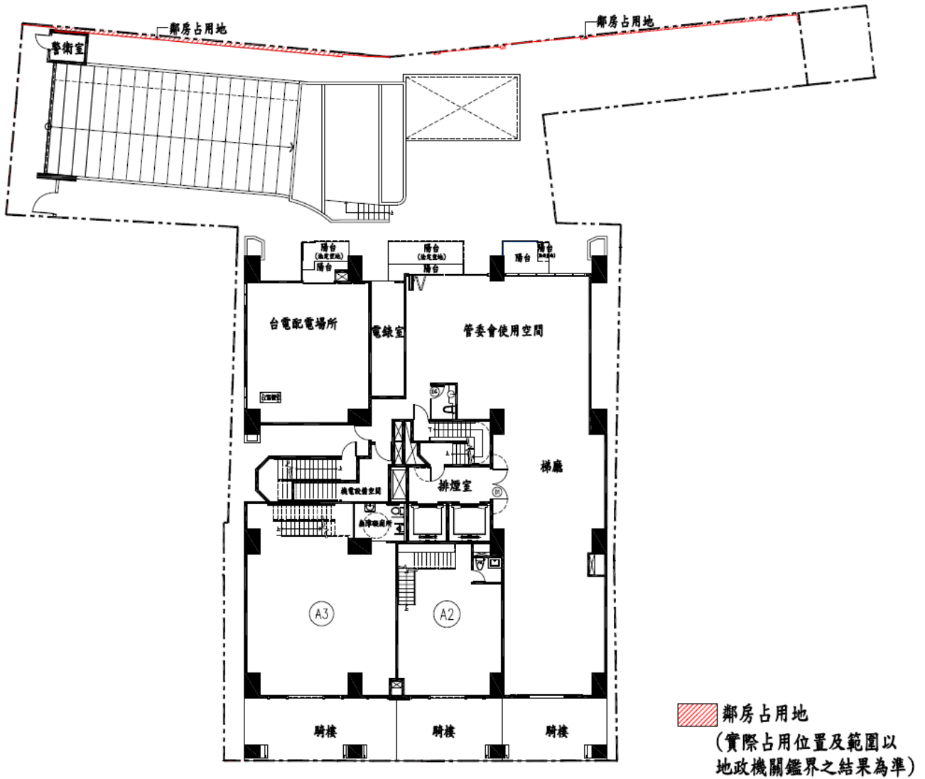
壹樓平面圖
