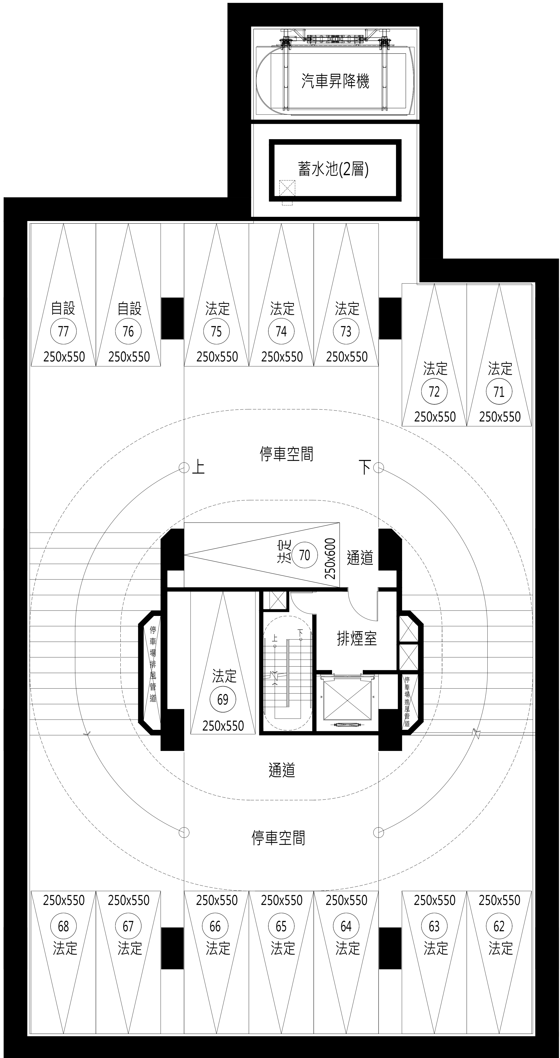
地下二層平面圖
