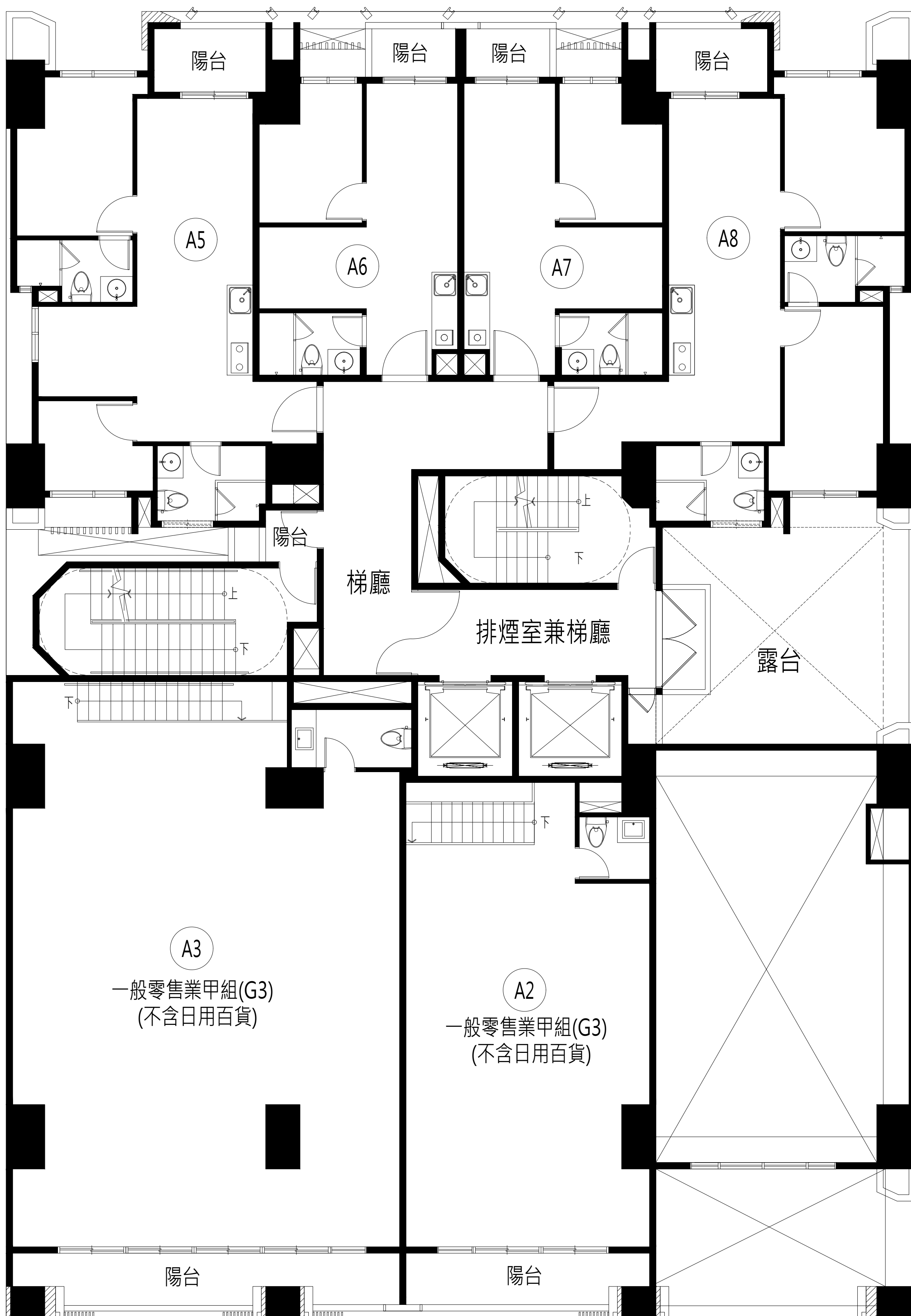
二樓平面圖
