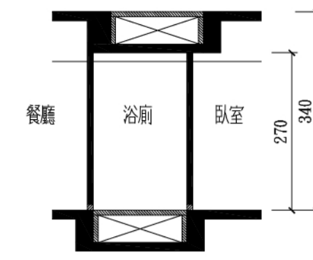
A5 戶浴廁樓層版區B剖面圖
