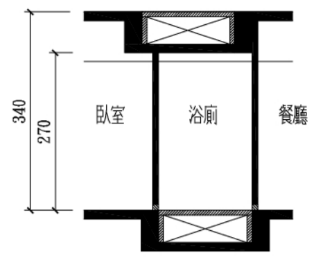
A6 戶浴廁樓層版區A剖面圖
