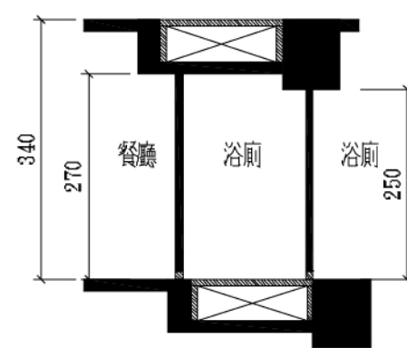
A4 戶浴廁複層版區D剖面圖
