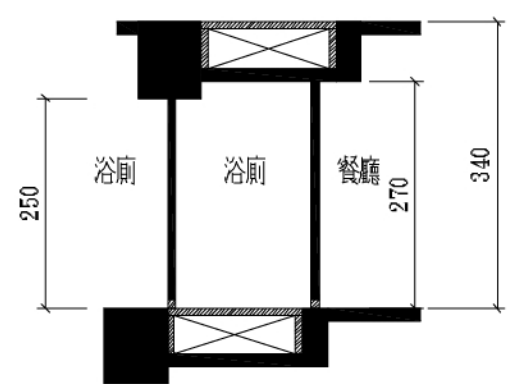
A7 戶浴廁複層版區A剖面圖
