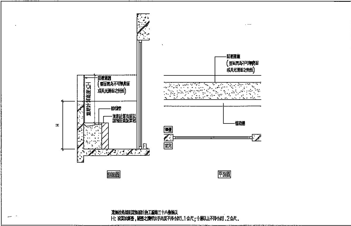
圖例二十一 陽臺內側設立固定傢俱台度增高
