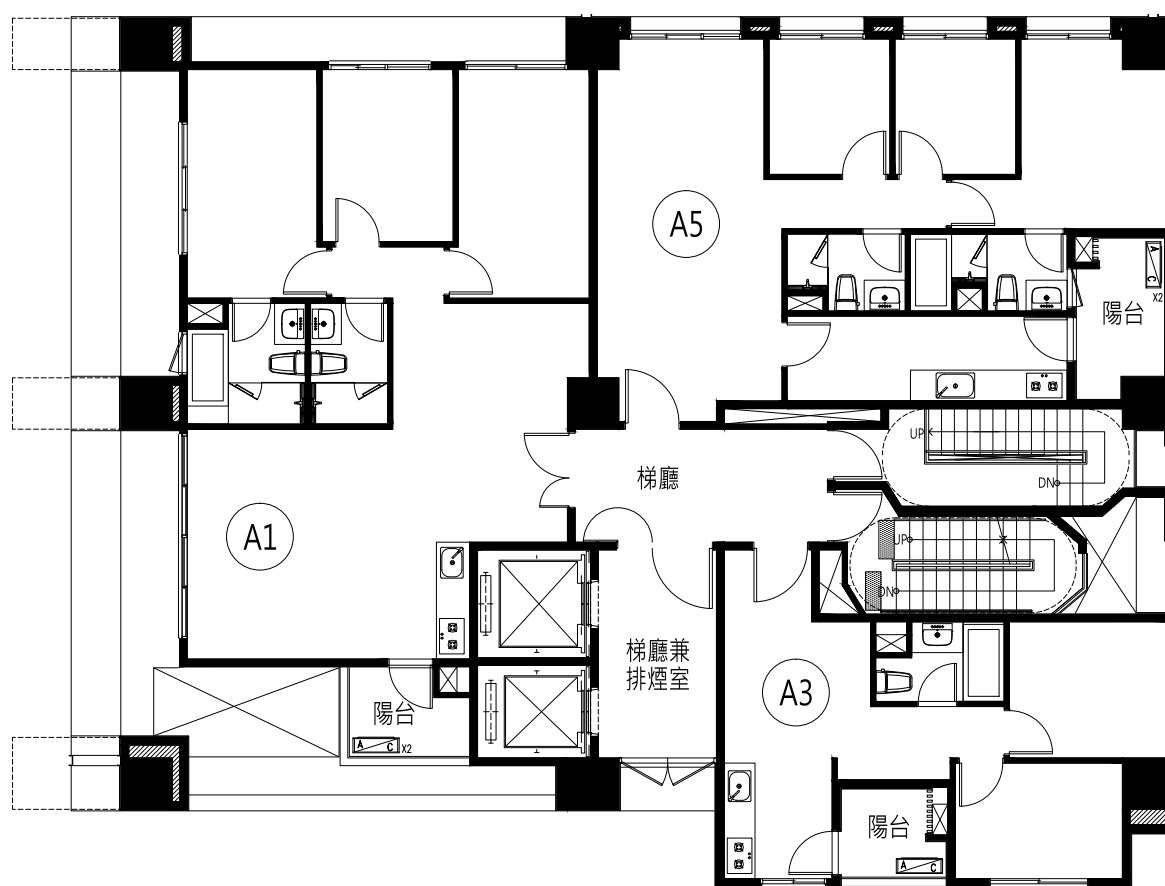
十四層平面圖
