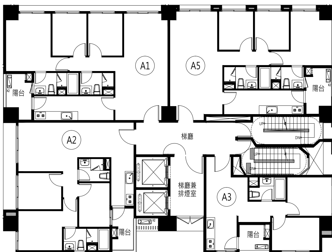
七~十層平面圖
