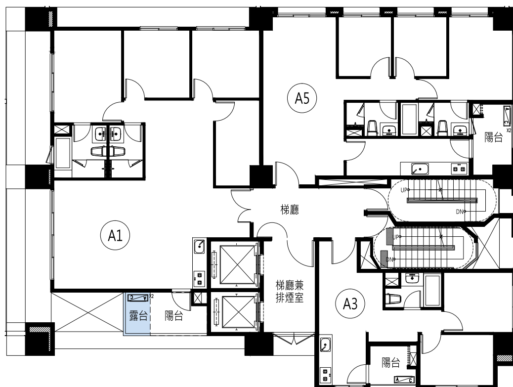
十二層平面圖
