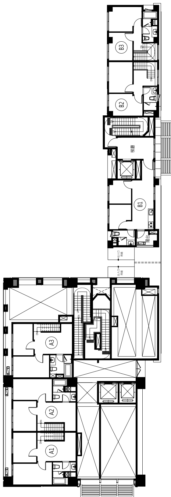
二層平面圖
