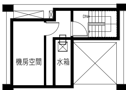
B棟 / 屋突三層平面圖
