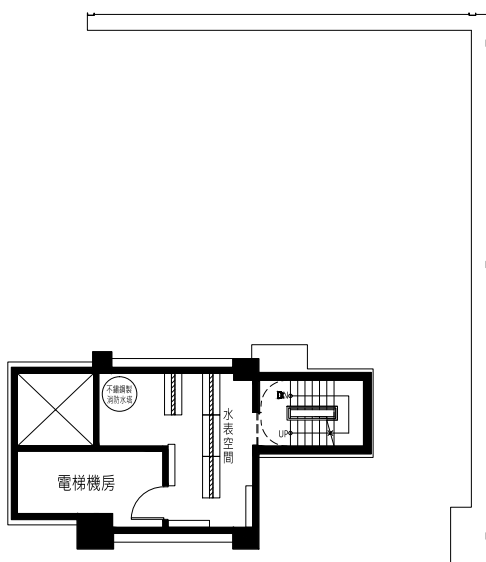
A棟 / 屋突二層平面圖
