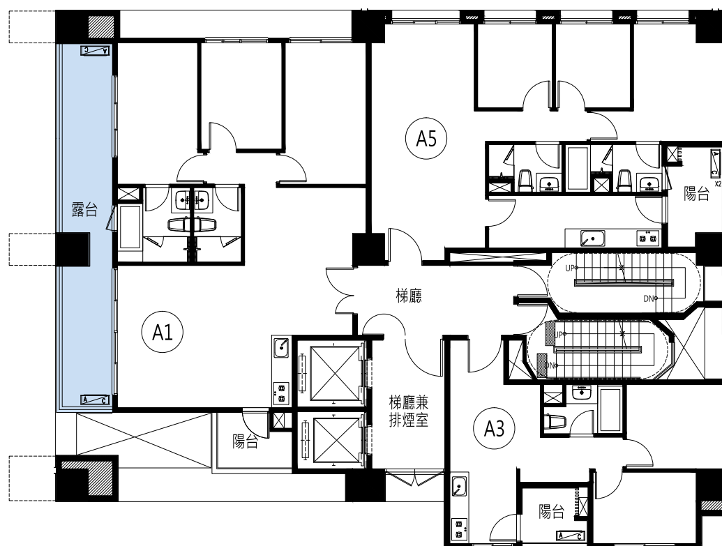
十三層平面圖
