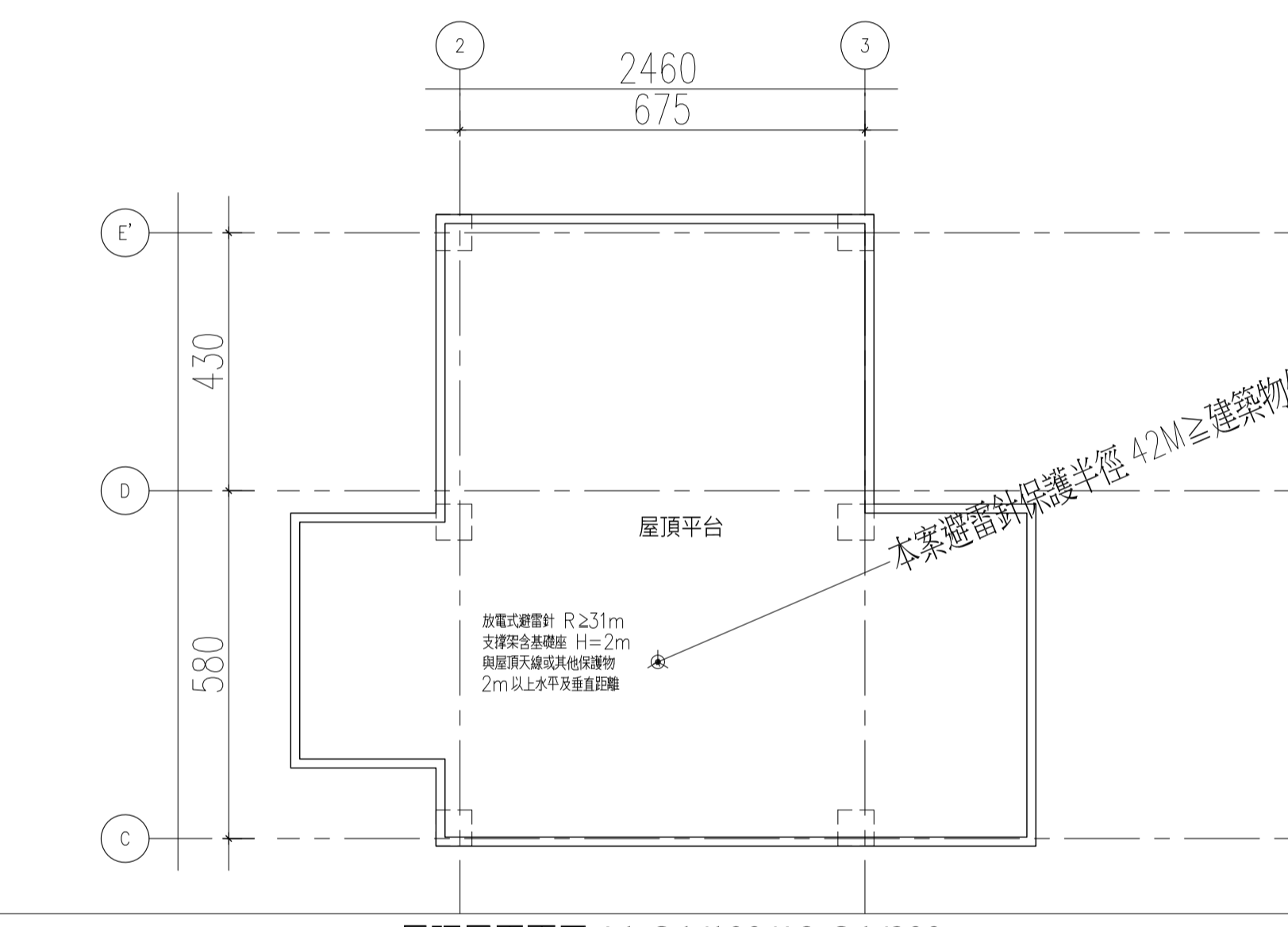
屋頂層平面圖 A1-S:1/100/A3-S:1/200
