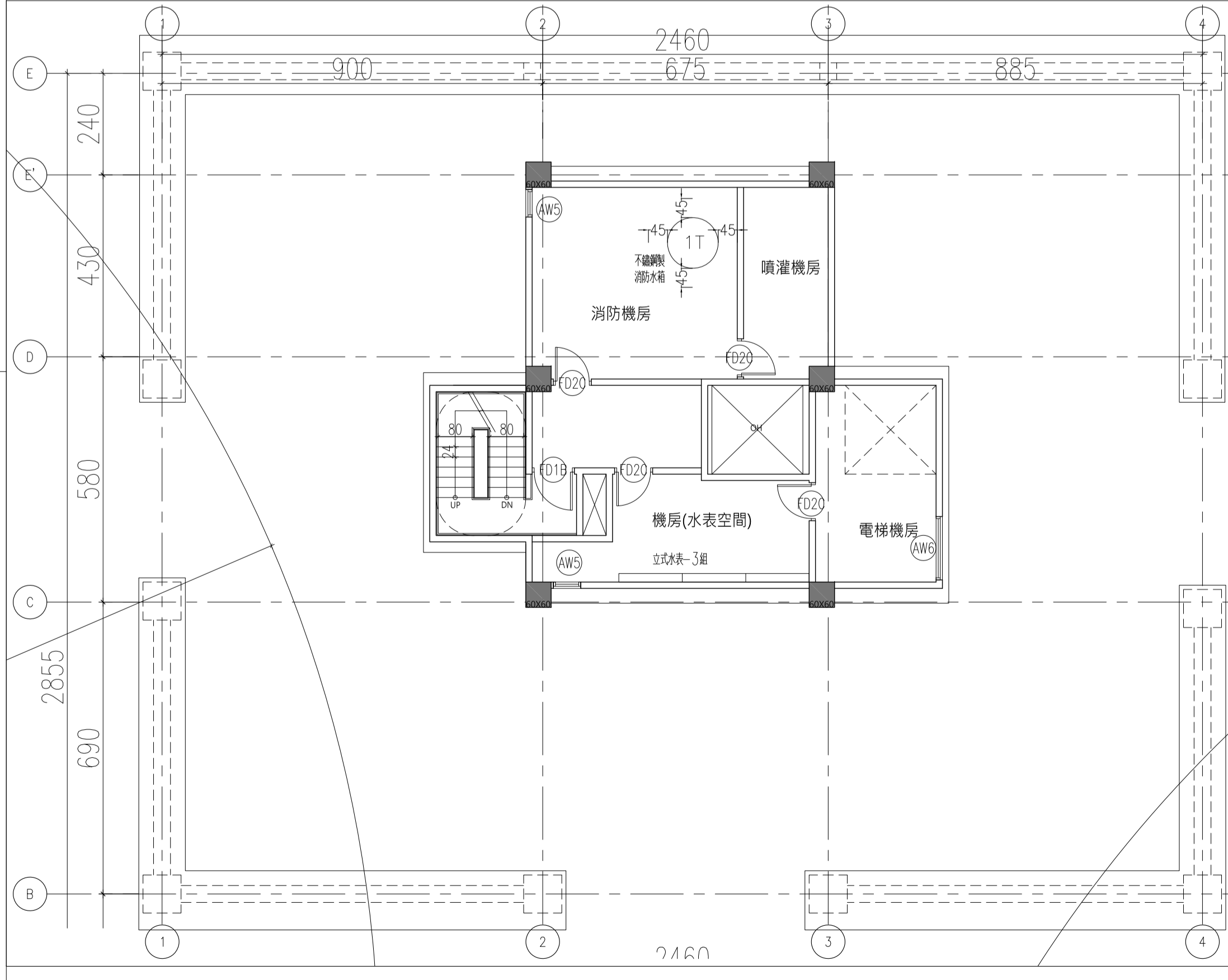
屋突二層平面圖 A1-S:1/100/A3-S:1/200
