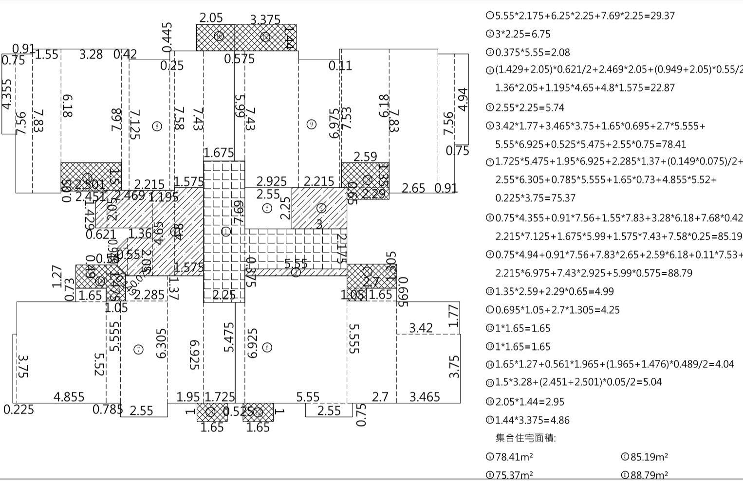
十四層面積計算示意圖 A1-S:1/200/A3-S:1/400
