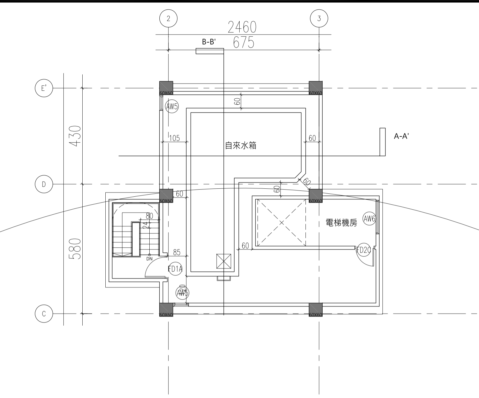
屋突三層平面圖 A1-S:1/100/A3-S:1/200
