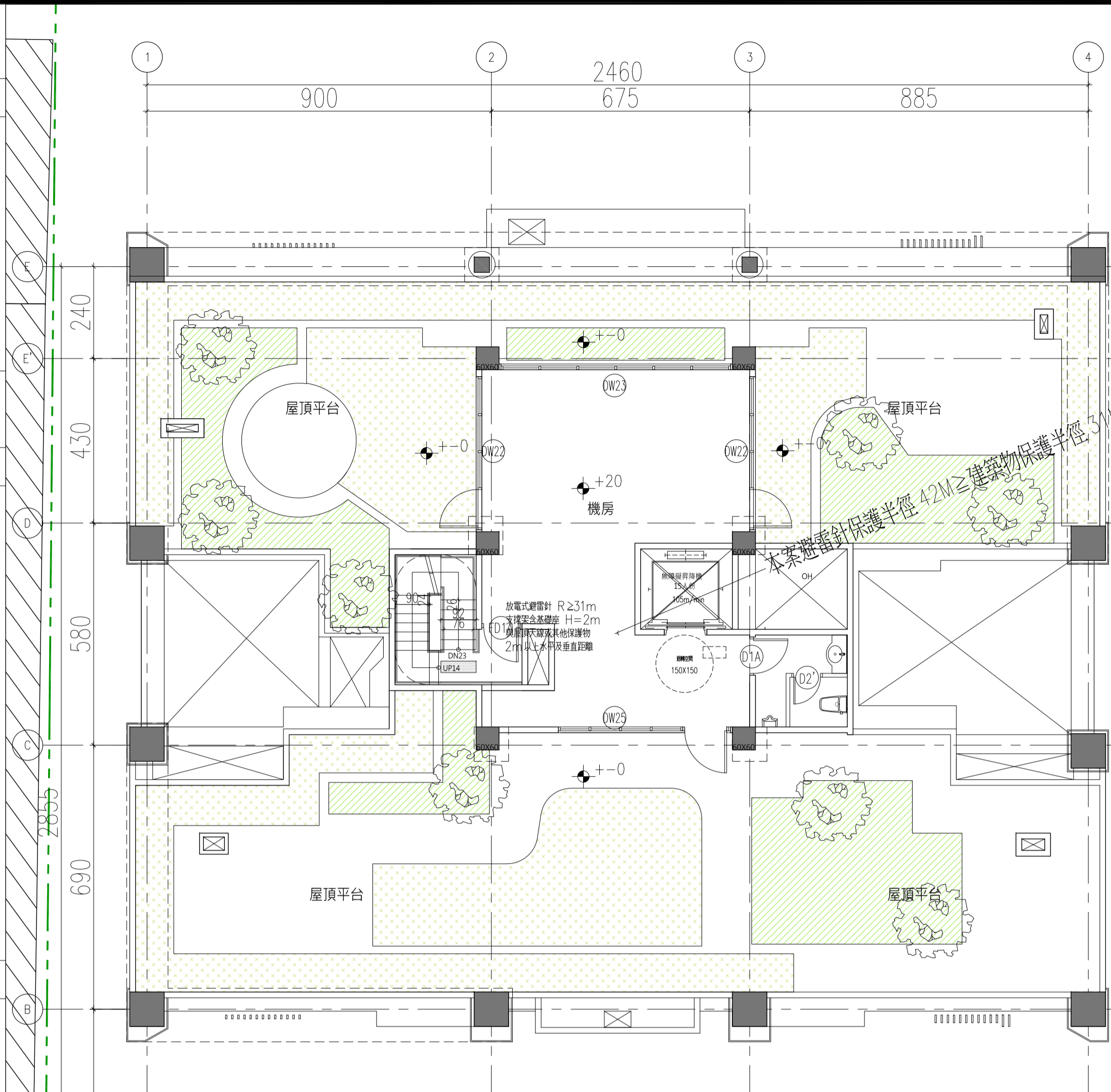
屋突一層平面圖 A1-S:1/100/A3-S:1/200
