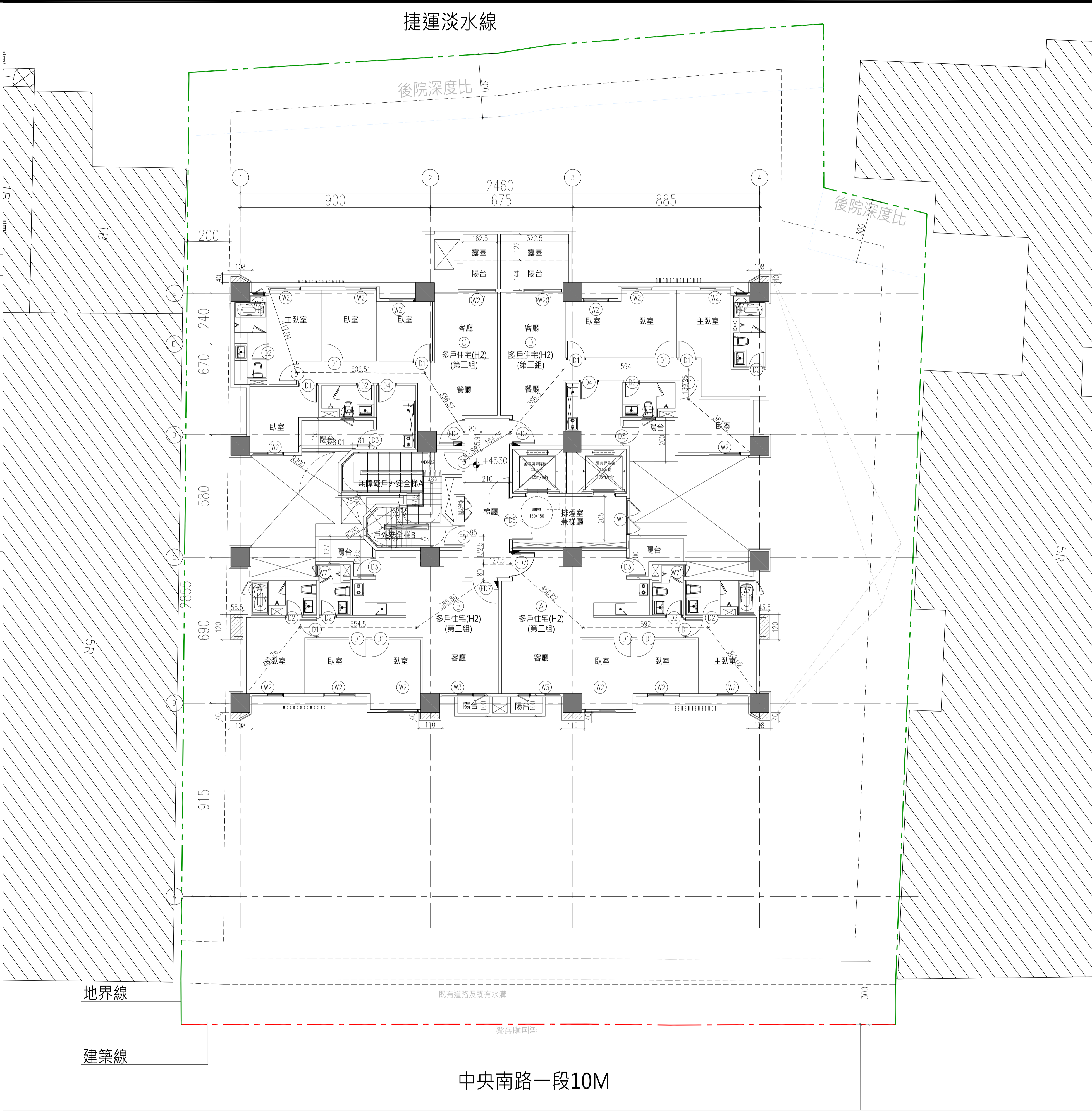
十四層平面圖 A1-S:1/100 A3-S1:200
