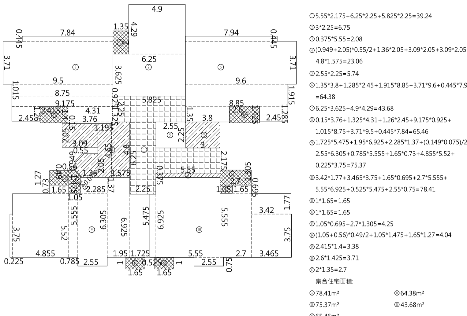
四層-十三層標準層面積計算示意圖 A1-S:1/200/A3-S:1/400
