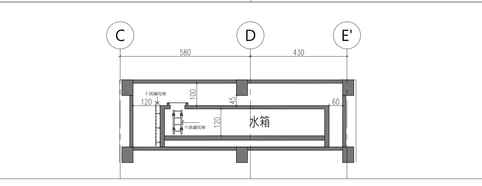
水箱剖面圖B-B' A1-S:1/100/A3-S:1/200
