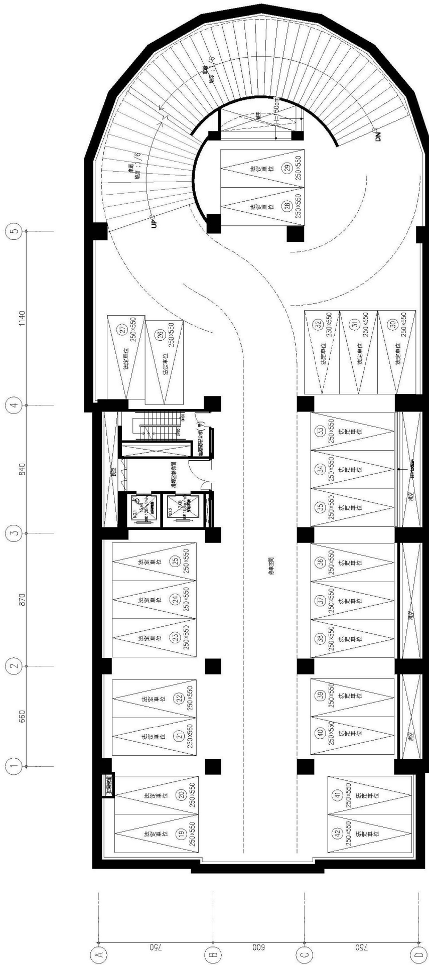
① 地下二層平面示意圖
