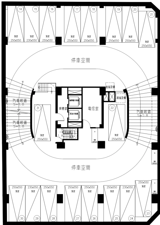
地下壹層平面圖
