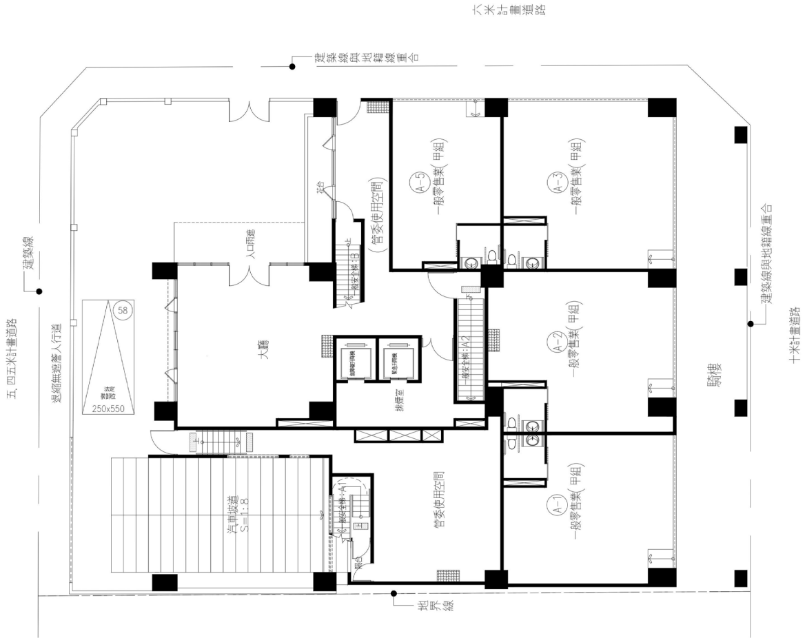
壹層平面圖
