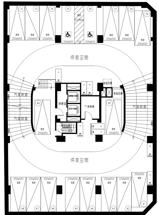
地下貳層平面圖
