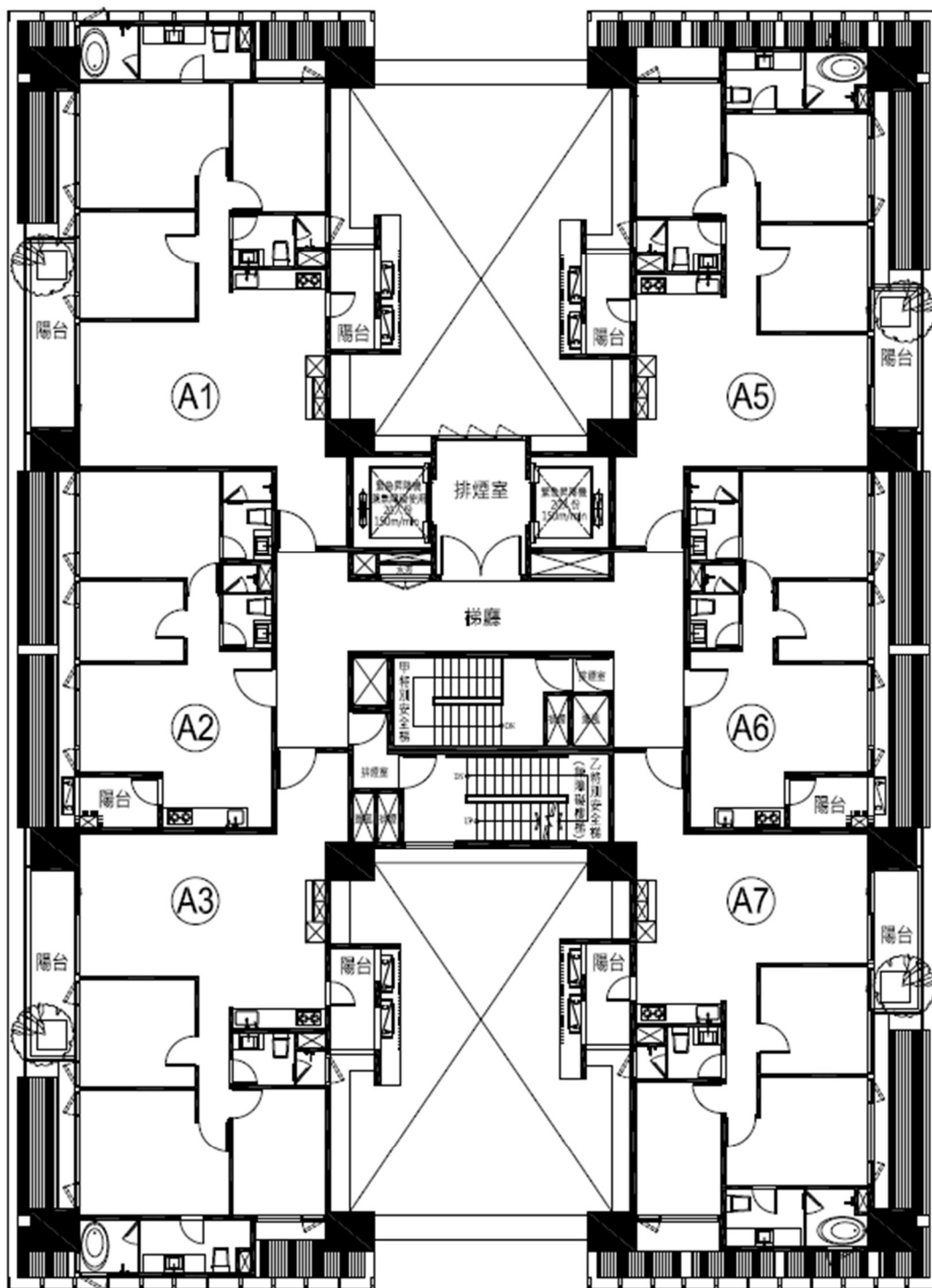
① 拾捌層平面圖
