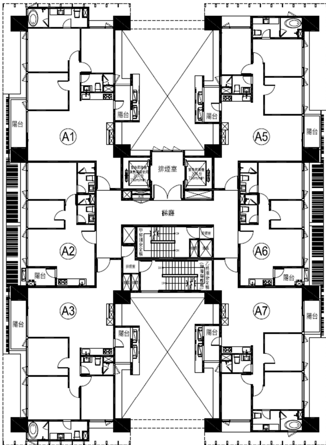
① 參~拾柒層平面圖(奇數層)
