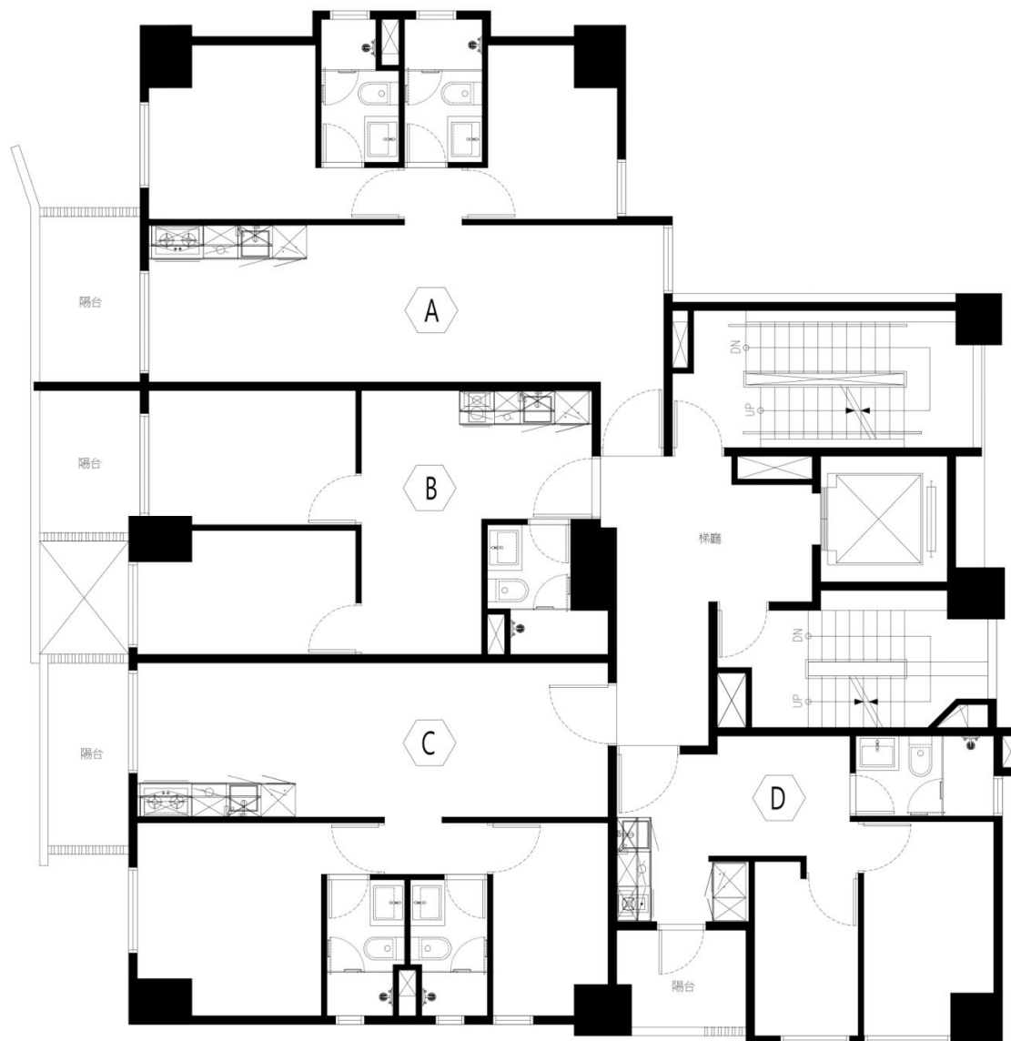
三至六層平面圖
