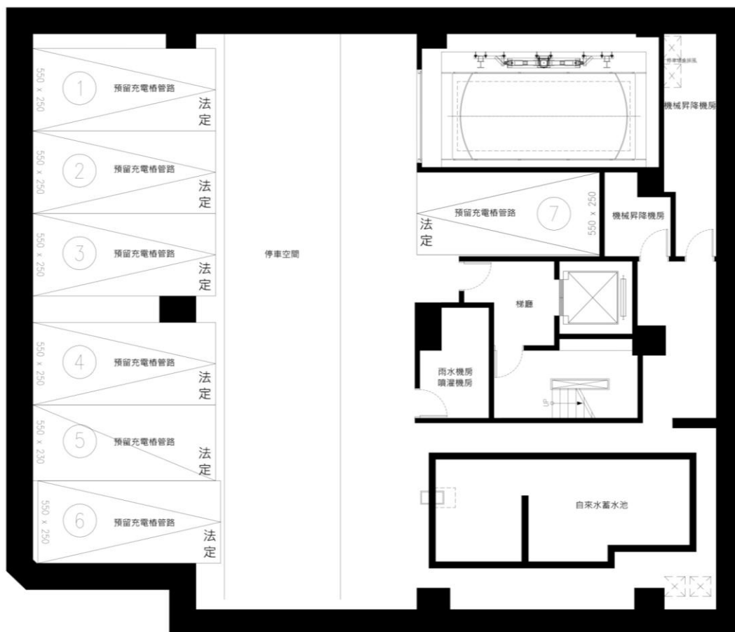
地下三層平面圖
