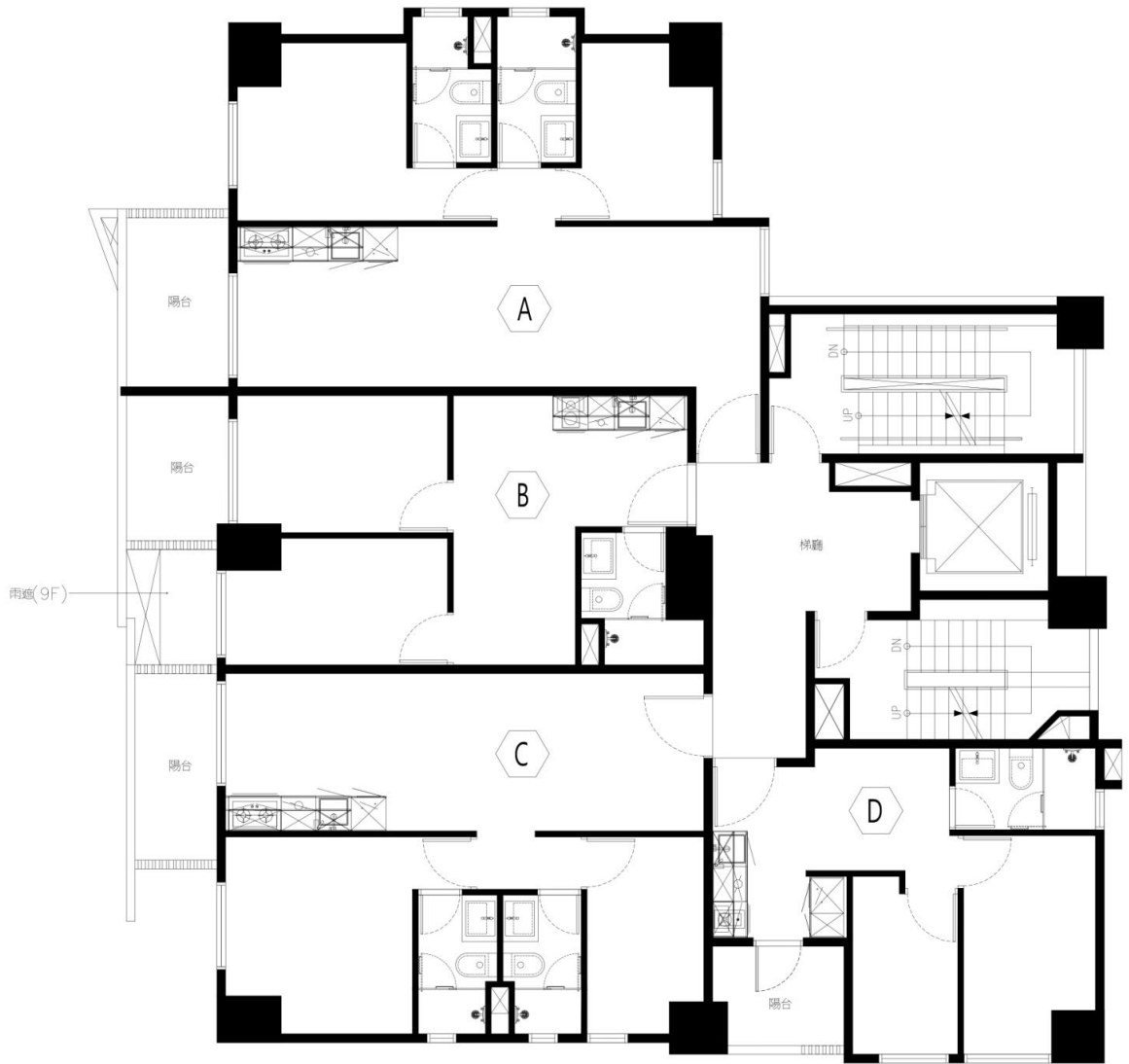
九至十一層平面圖
