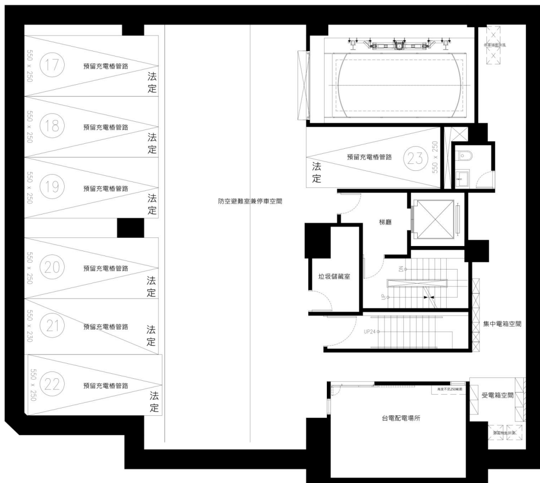
地下一層平面圖
