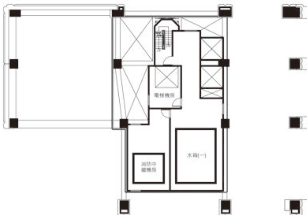
屋突一平面圖
