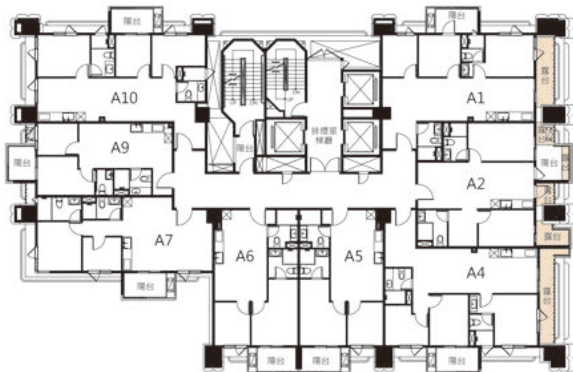
二十一層平面圖
