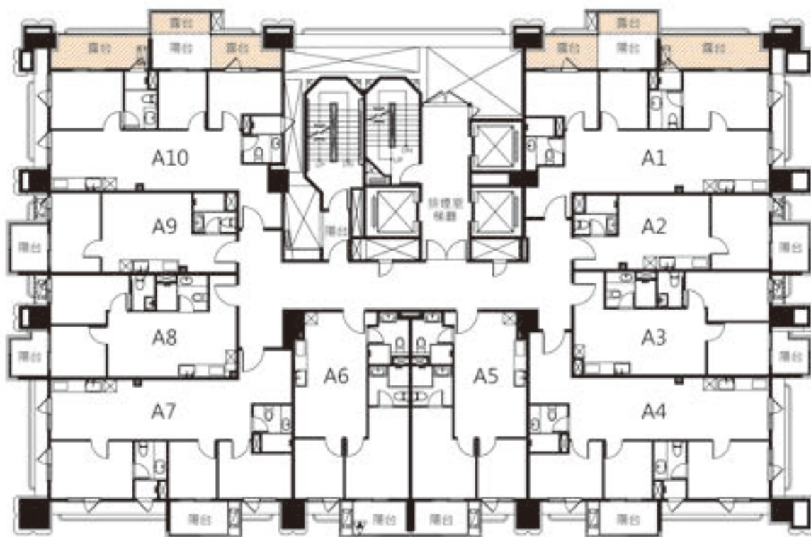
七層平面圖
