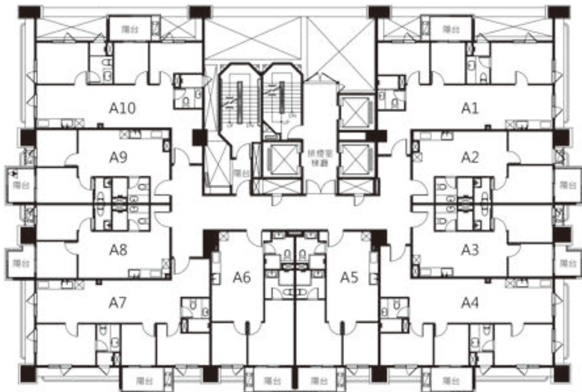
五層平面圖
