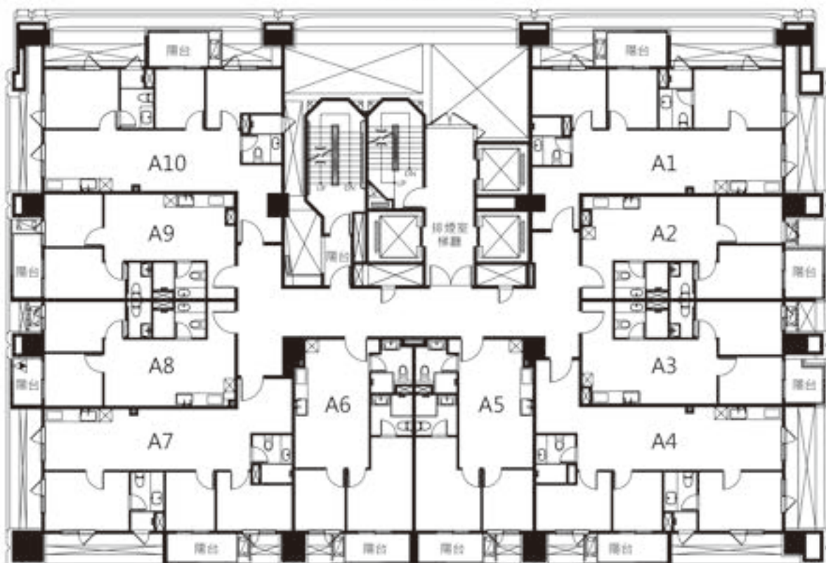
五層平面圖
