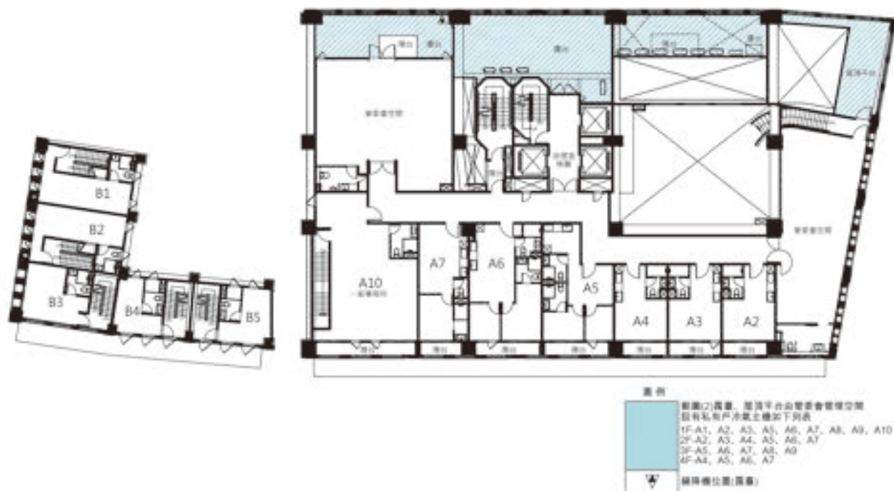
二層平面圖
