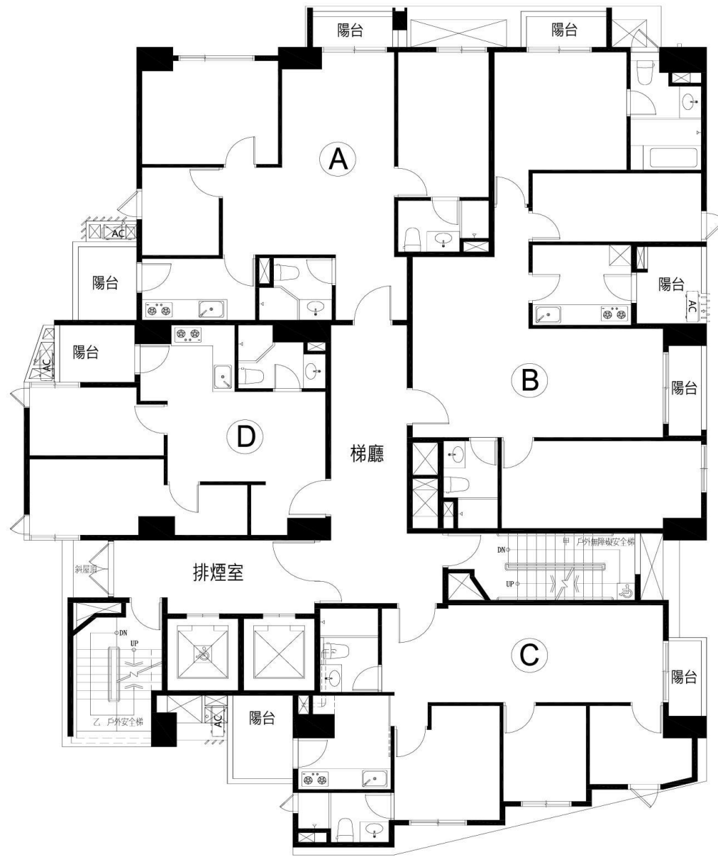
二層平面圖
