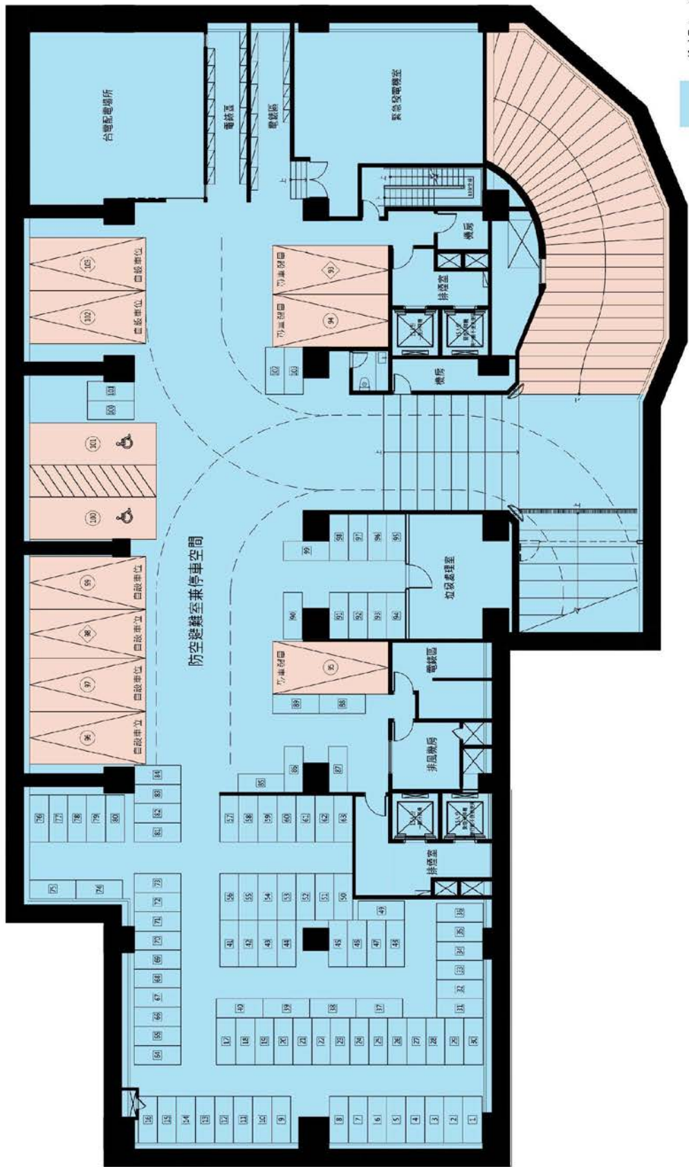
地下一層平面圖
