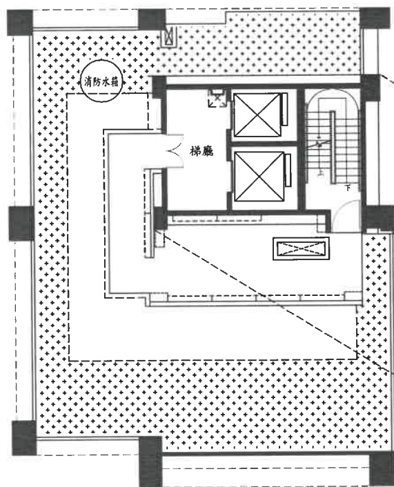
屋突一層平面圖
