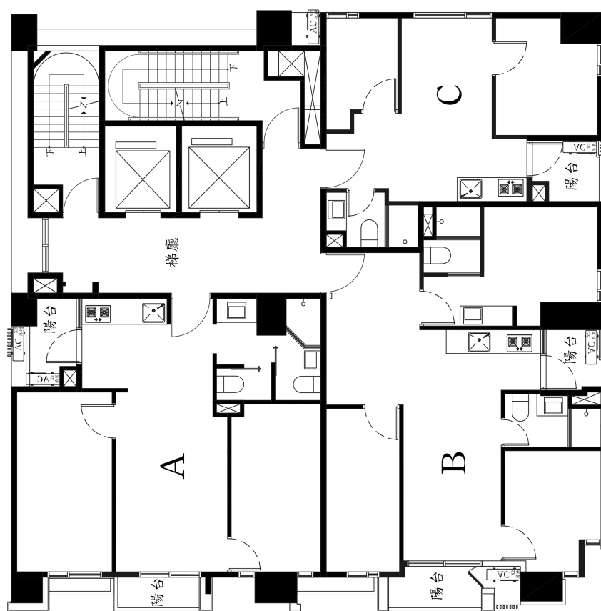
八層平面圖
