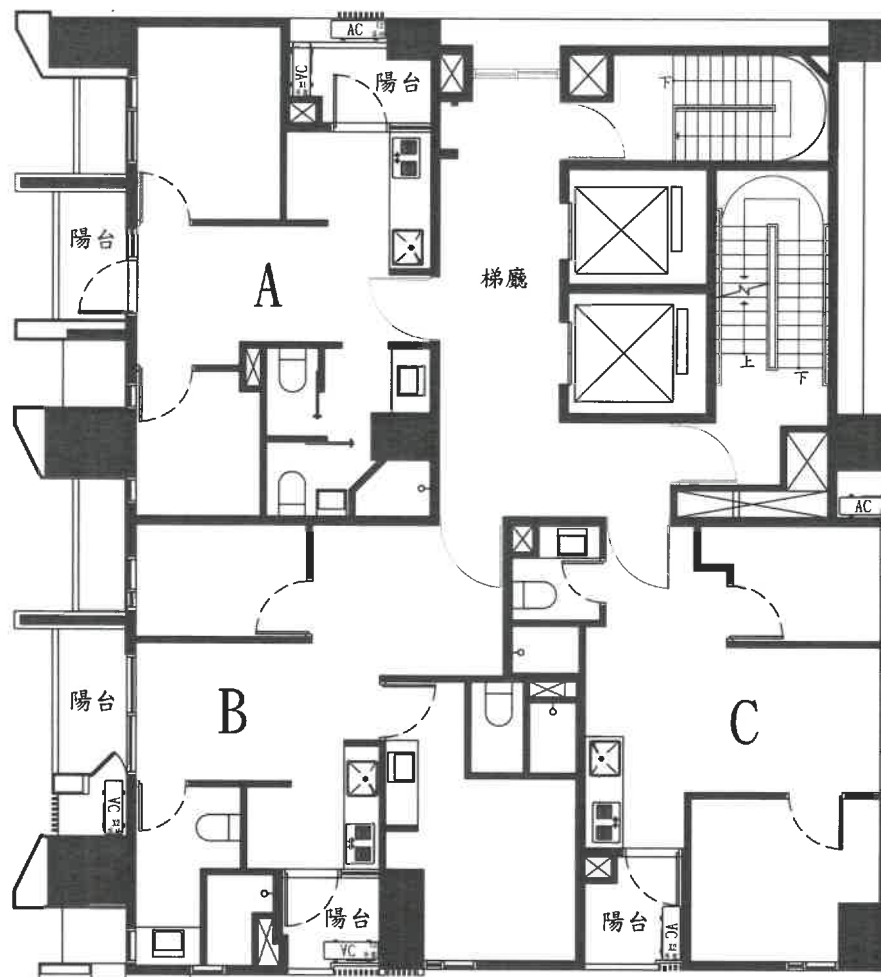
十二層平面圖
