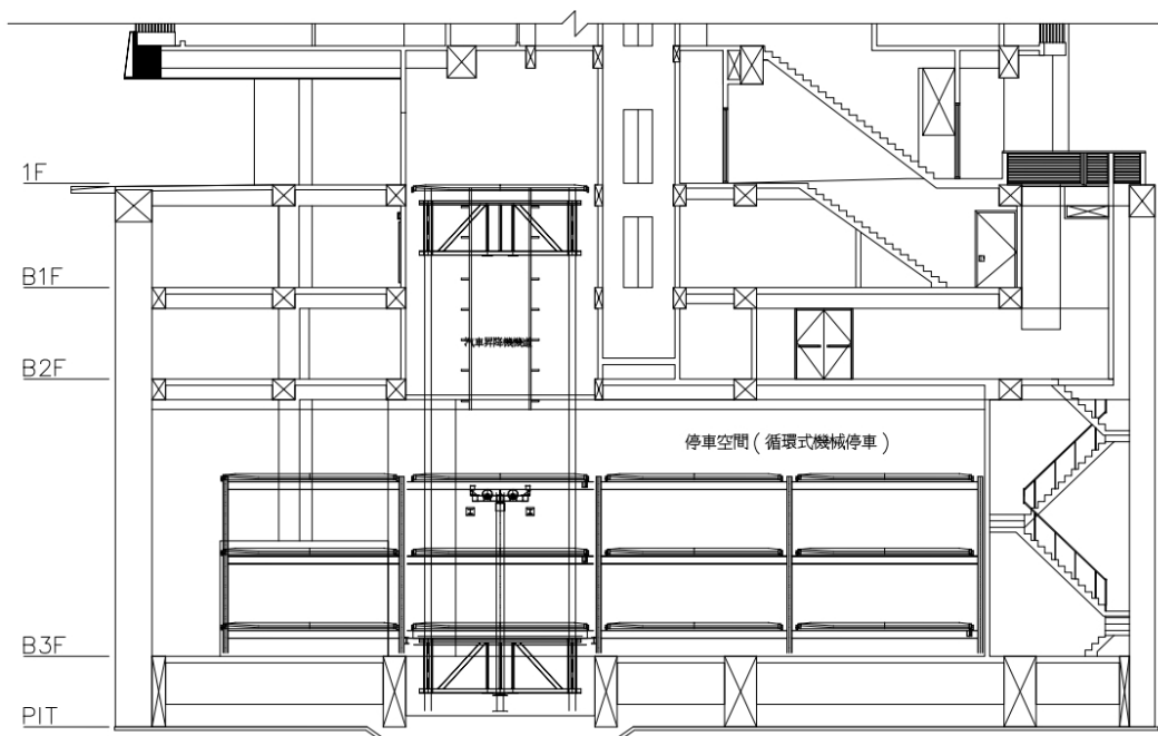
停車空間剖面圖
