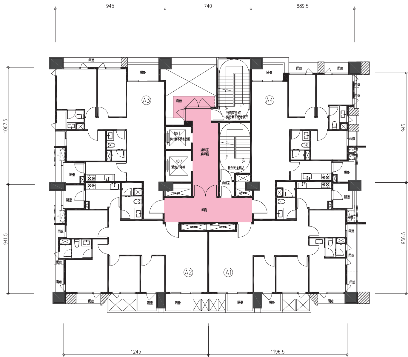
十六層平面圖
