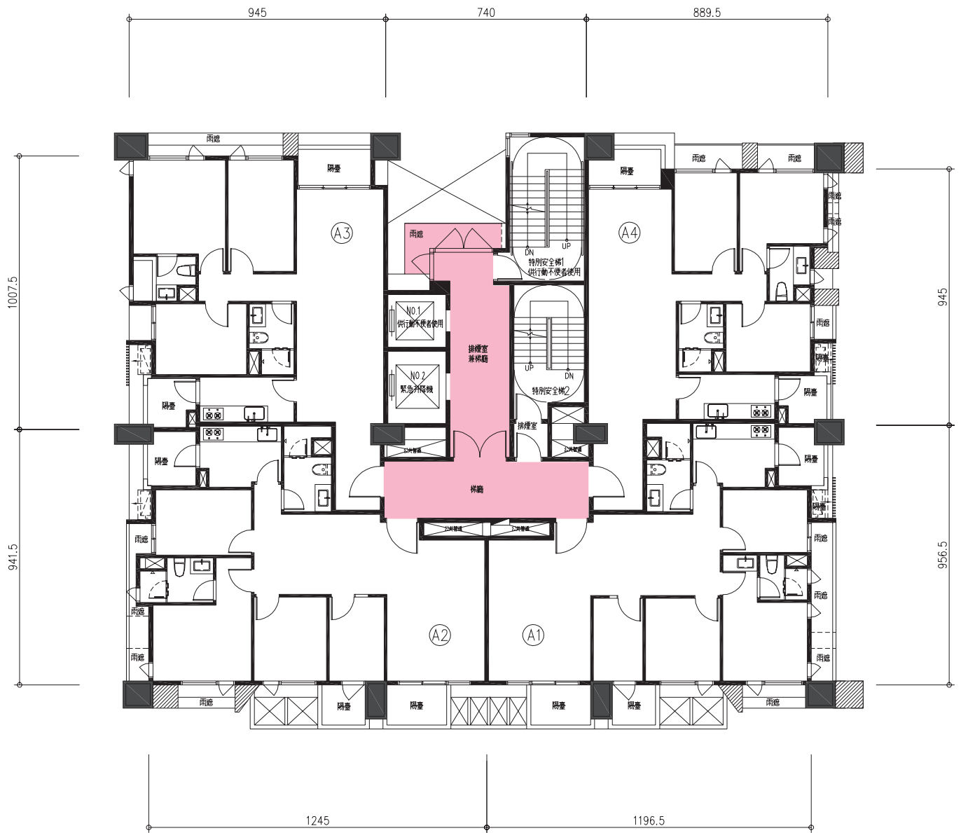
十七層平面圖
