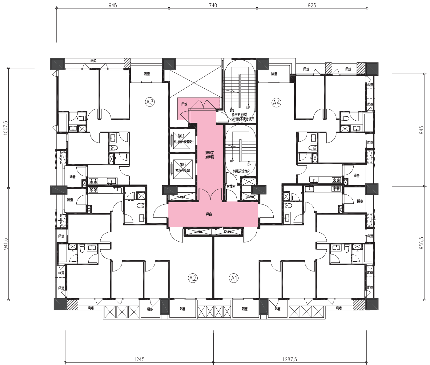
三層平面圖
