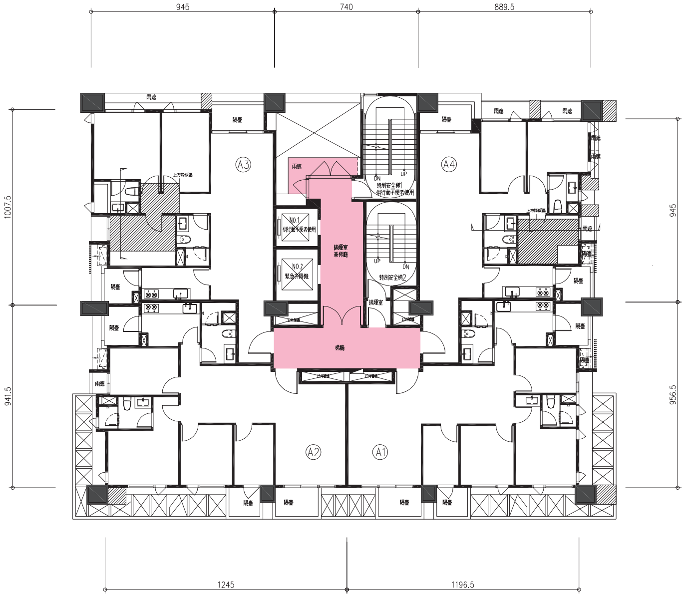
十八層平面圖
