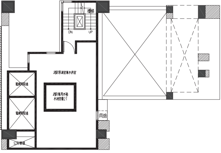
屋突二層平面圖
