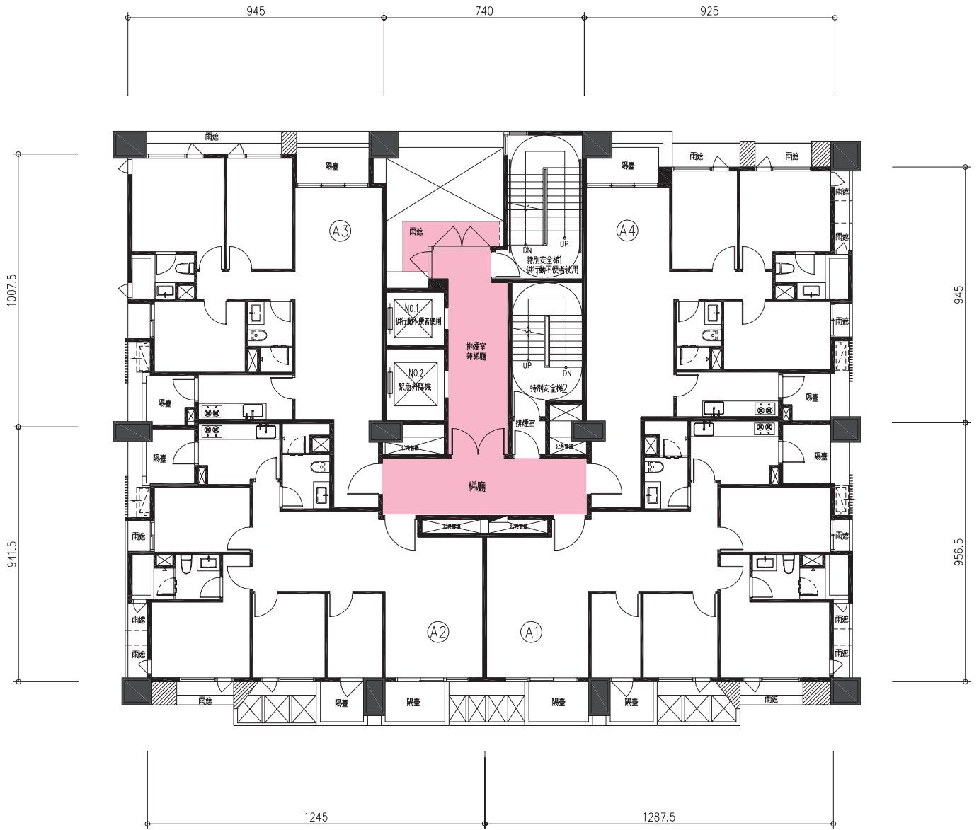
四層平面圖
